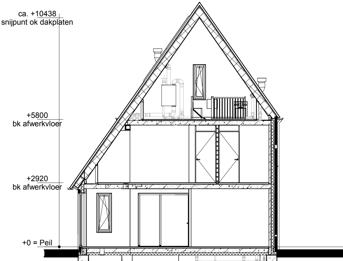
Doorsnede B2
