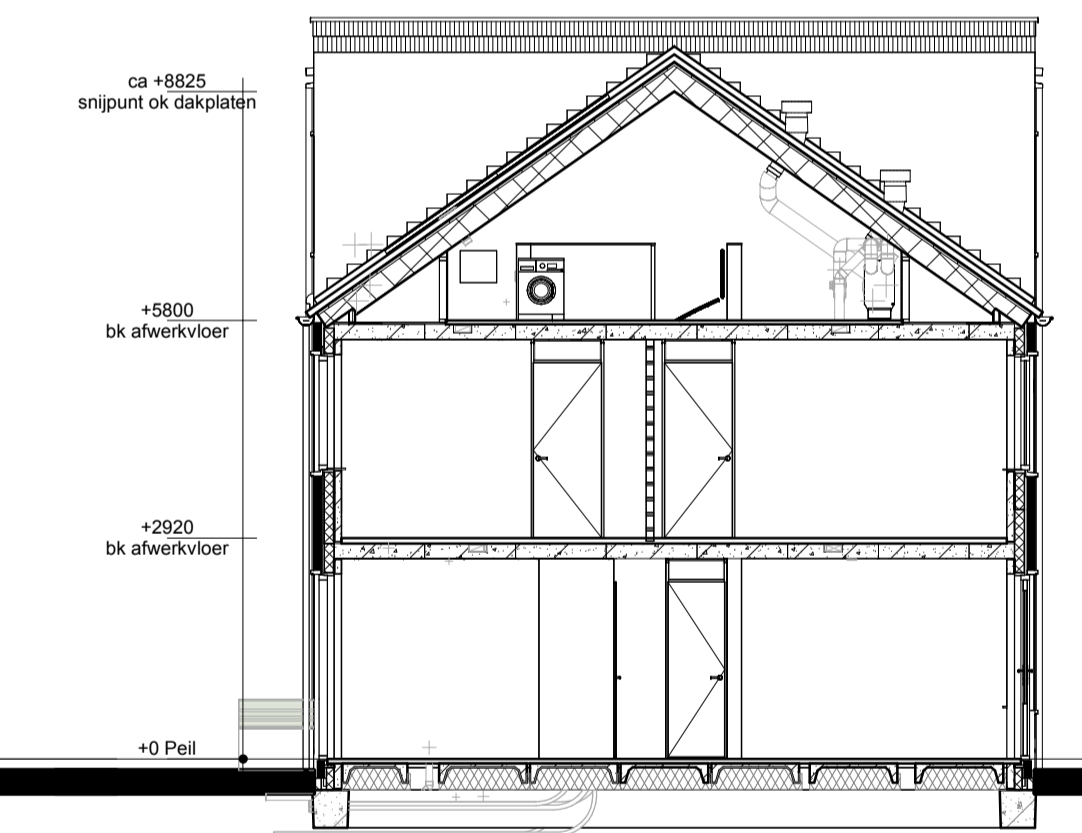
Doorsnede C1-C1
