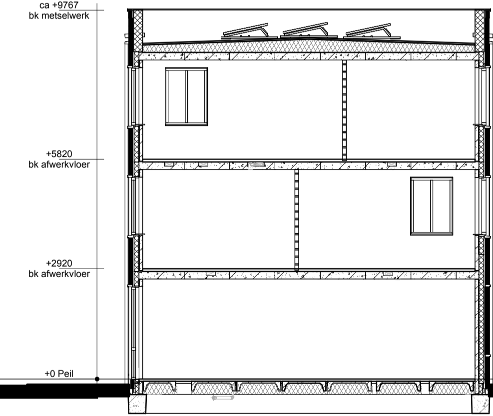
Doorsnede A1-A1
