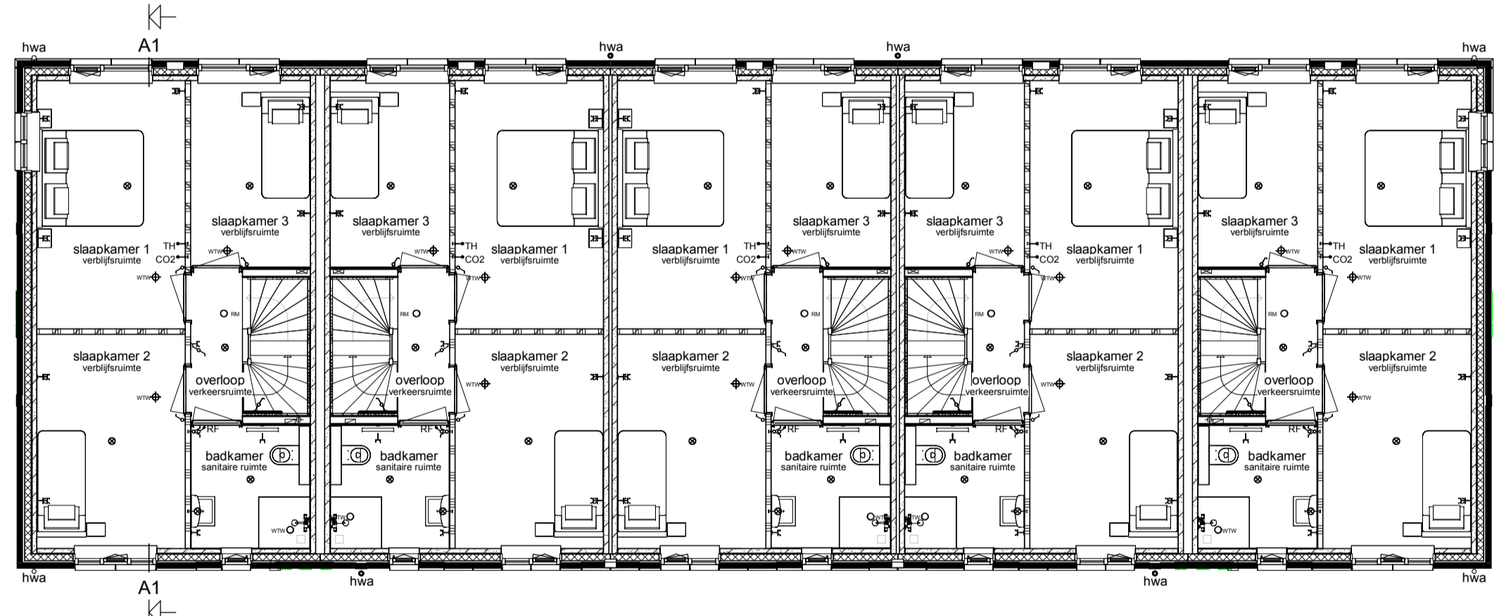
Begane grond
