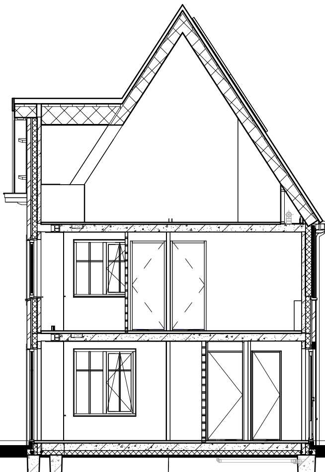
Doorsnede BB
