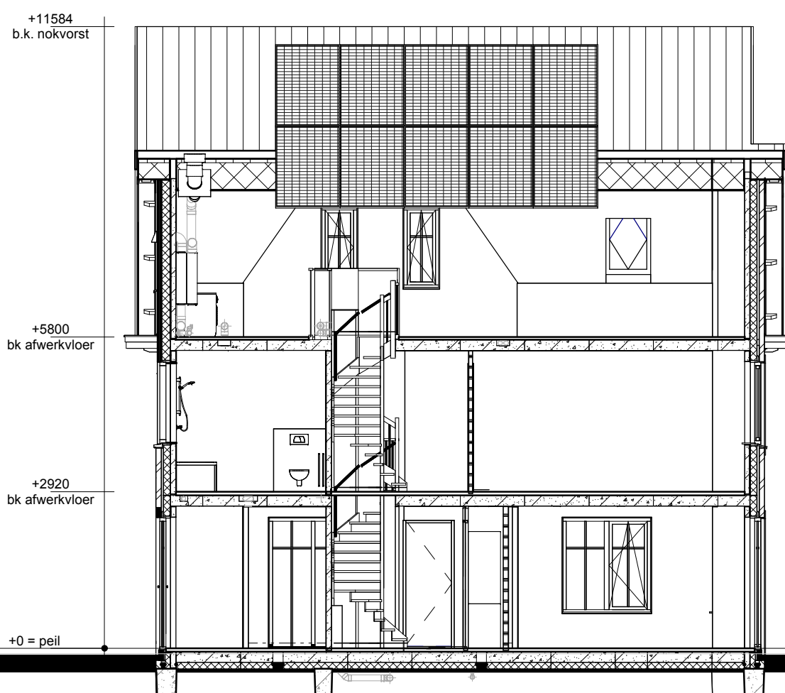
Doorsnede AA
