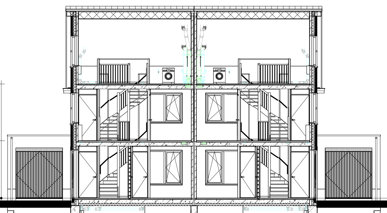
Doorsnede B1-B1
