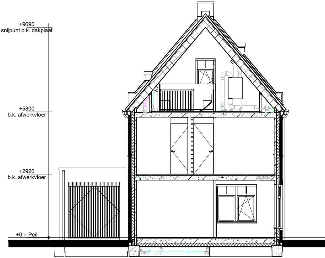
Doorsnede B2-B2
