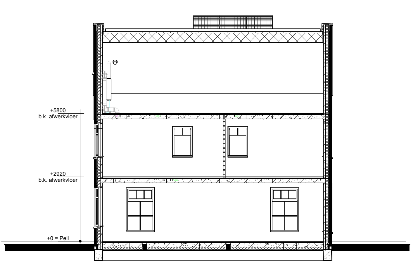
Doorsnede A2-A2
