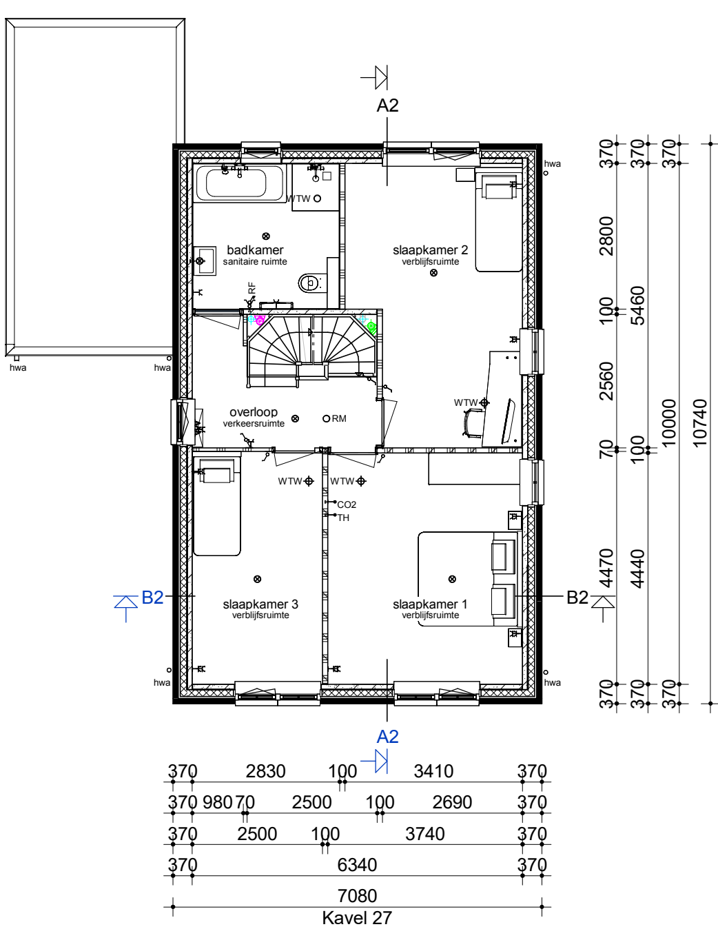
Verdieping
