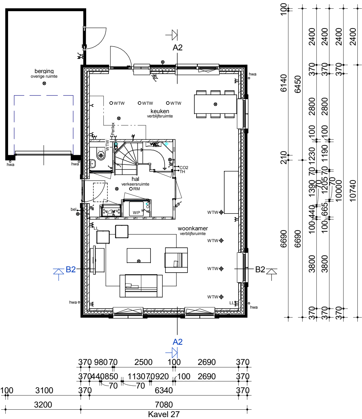
Begane grond
