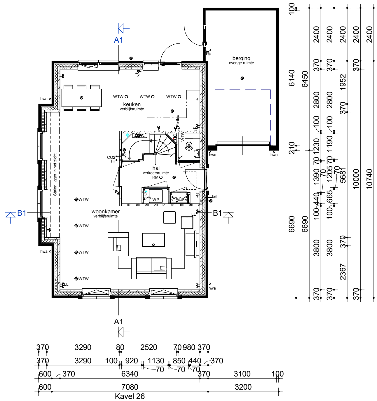
Begane grond
