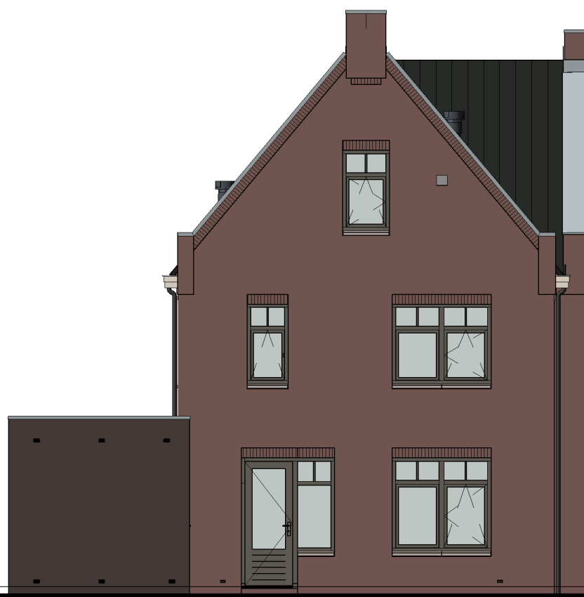
Kavel 26 Achtergevel
