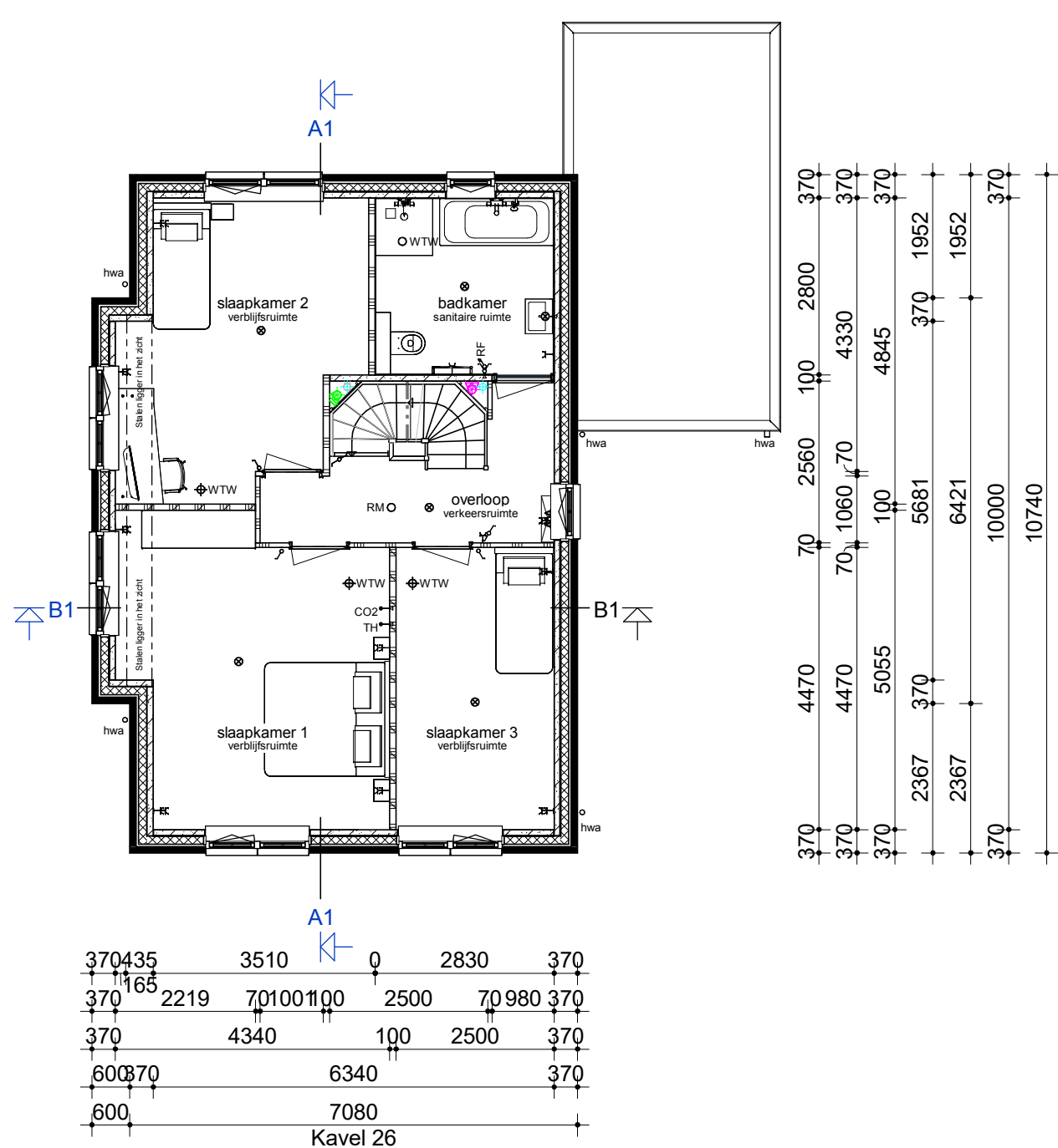
Verdieping
