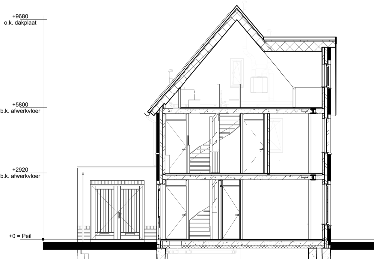
Doorsnede A-A
