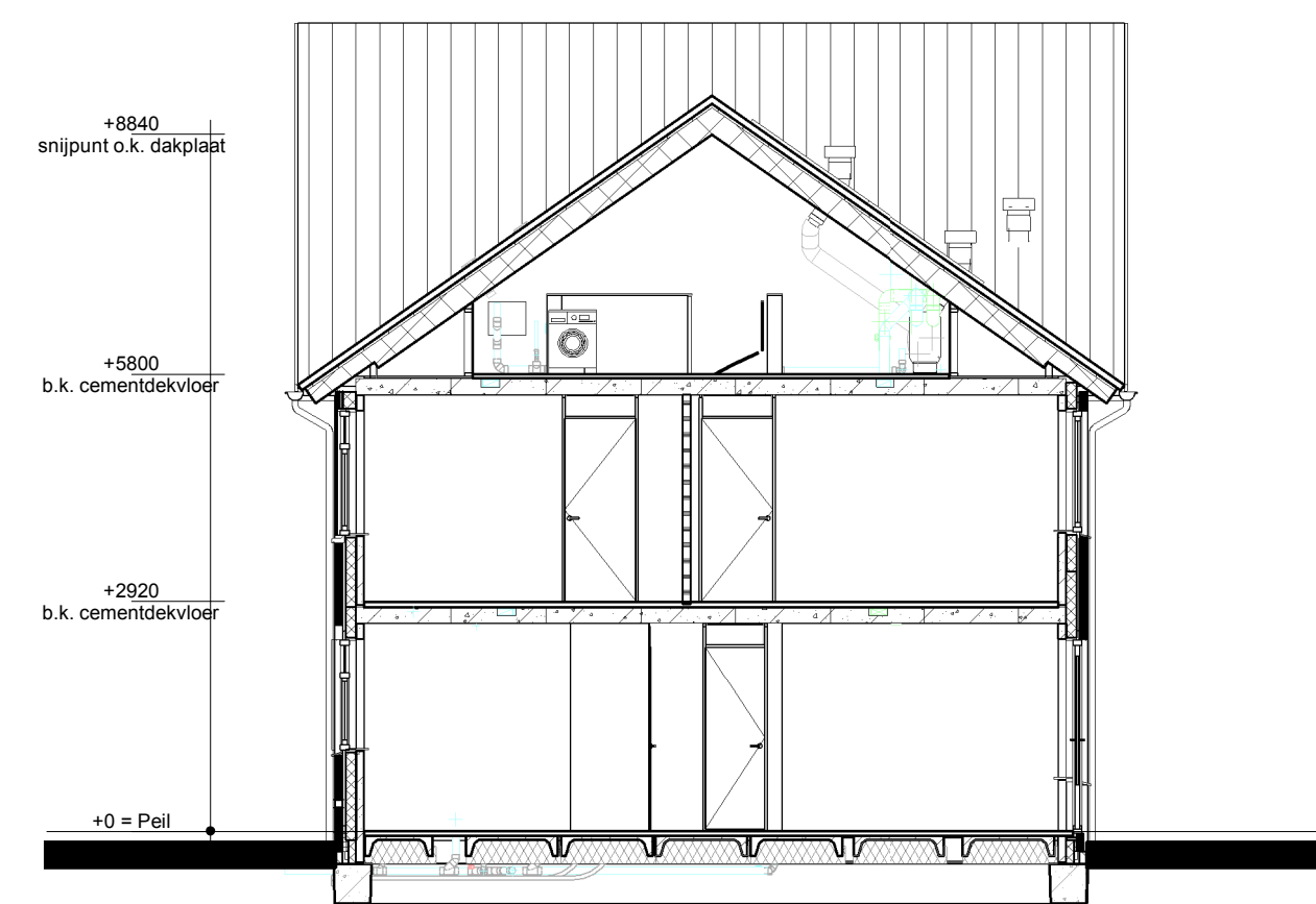
Doorsnede C1-C1
