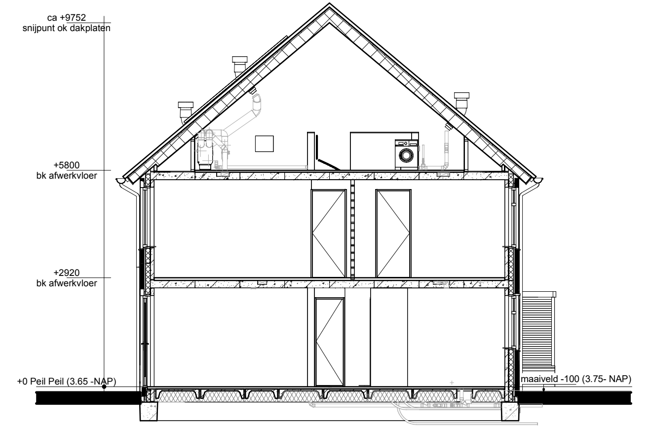
Doorsnede A1-A1
