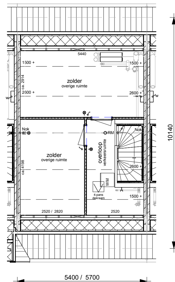
Optie 0567: scheidingswand op zolder
