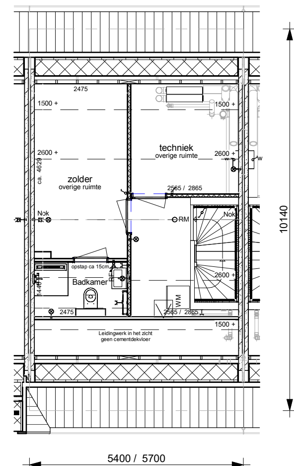
Optie : badkamer op zolder en extra zolderruimte
