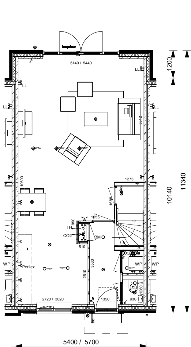
Optie 0305: 1200mm verlenging
