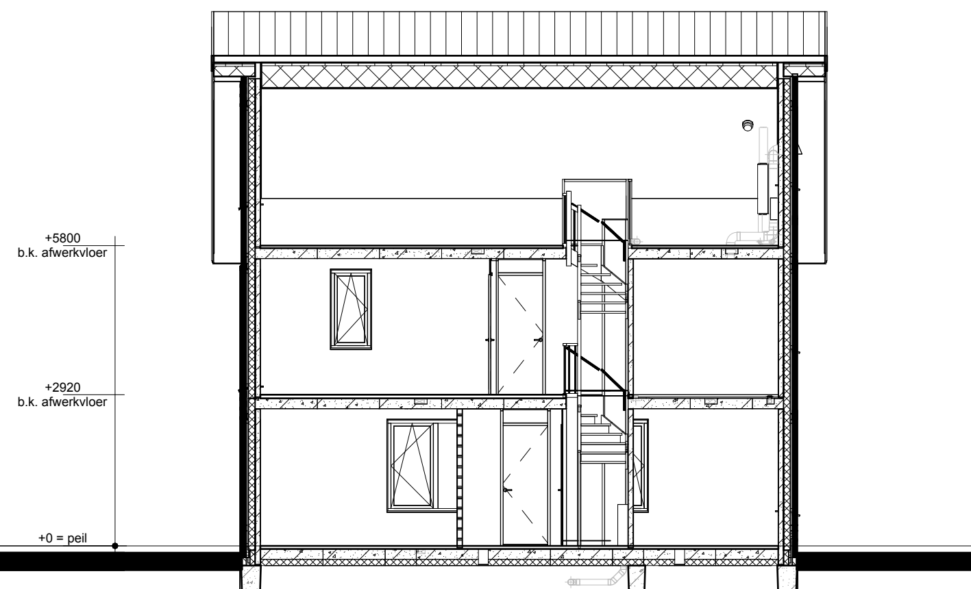
Doorsnede A1-A1
