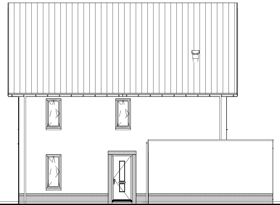
Kavel 01 & 08 Rechter zijgevel
