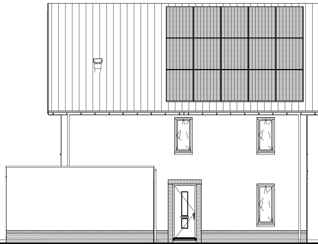
Linker zijgevel
