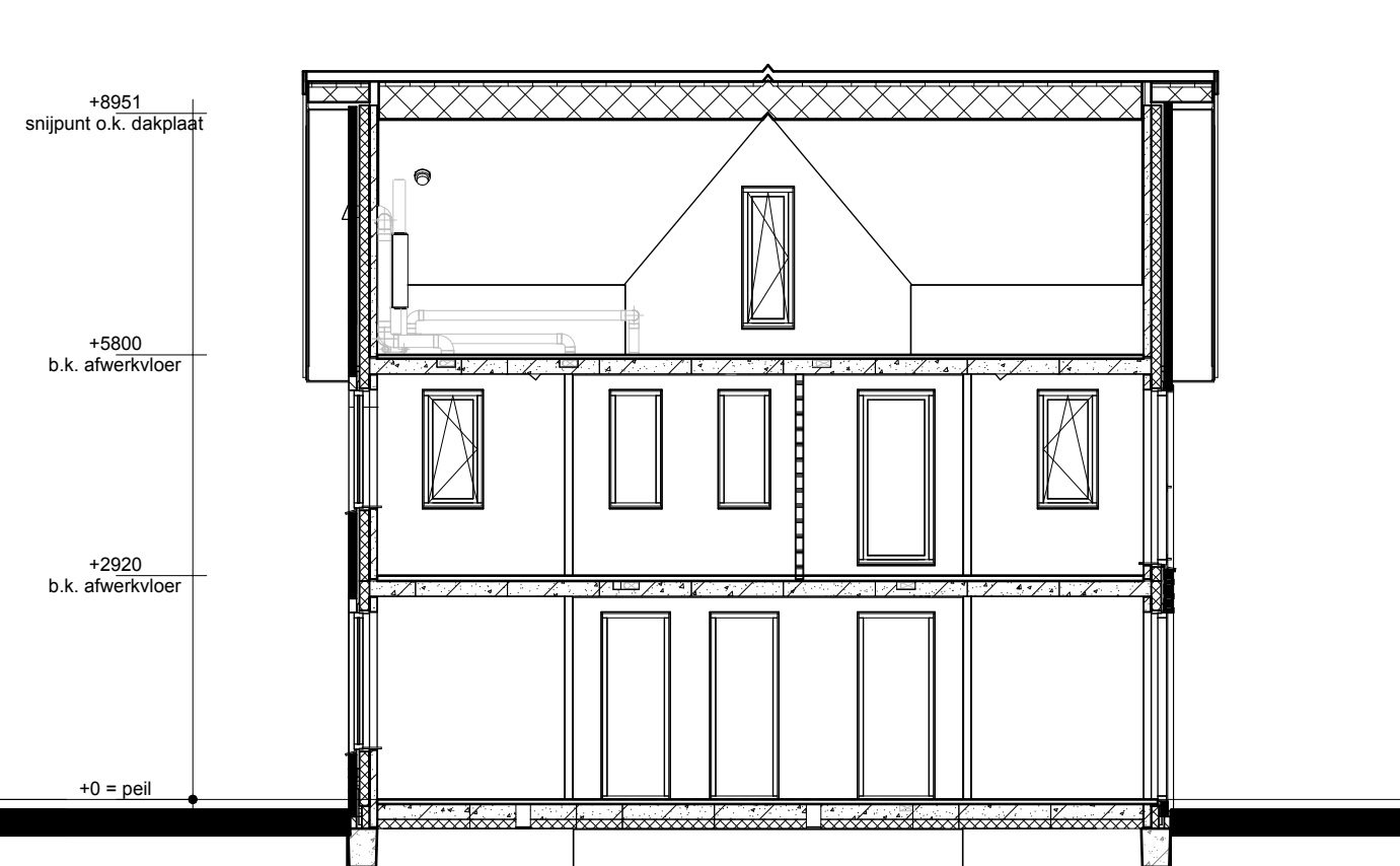
Doorsnede A3-A3
