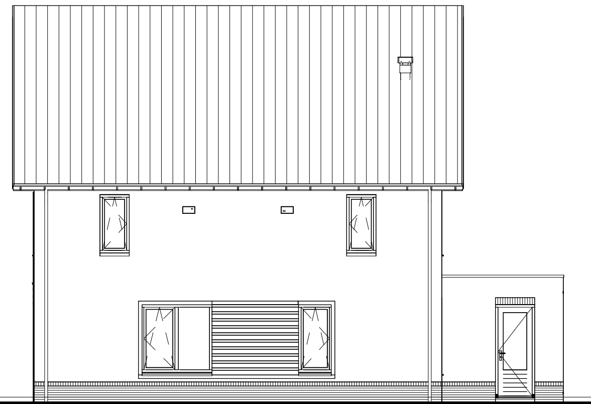
Rechter zijgevel
