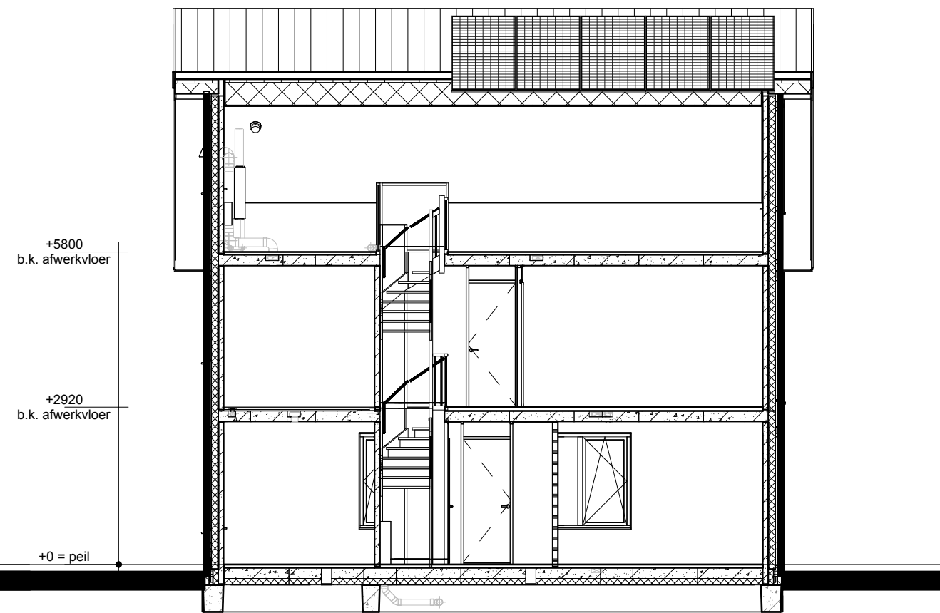
Doorsnede A6-A6
