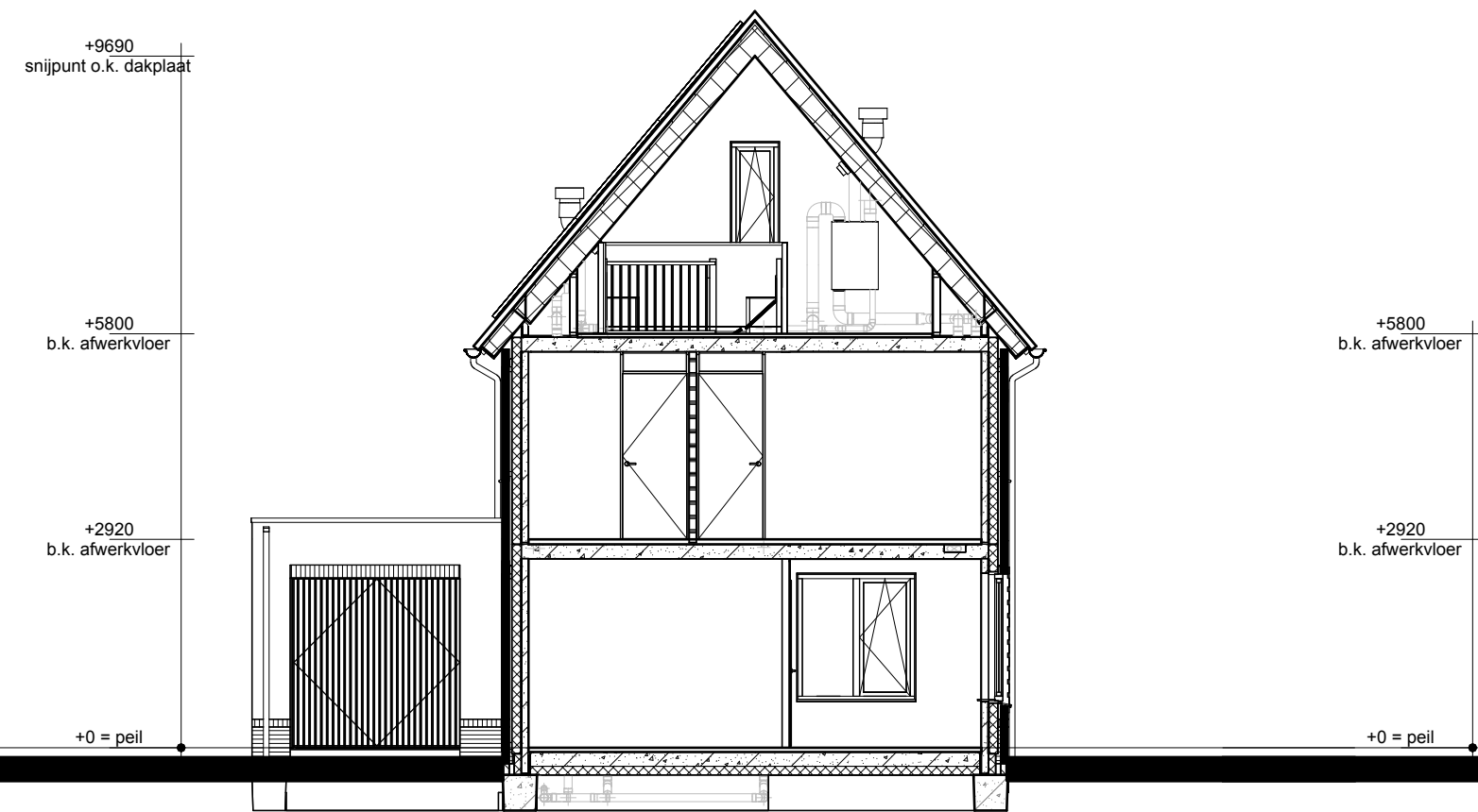
Doorsnede B6-B6
