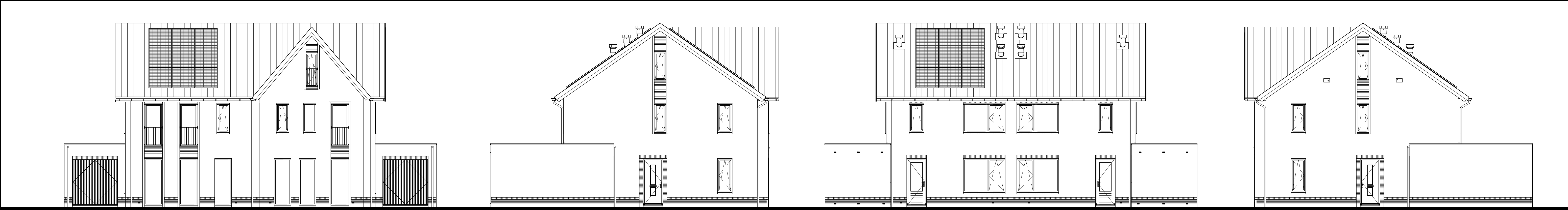
Voorgevel Kavel 06 Kavel 07 Linker zijgevel Kavel 06 Kavel 07 Achtergevel Kavel 06 Kavel 07 Rechter zijgevel Kavel 07
