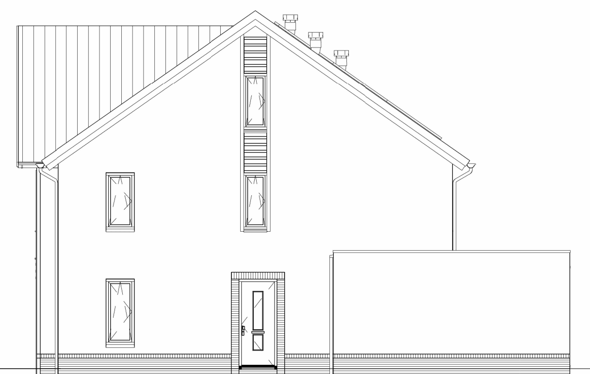
Rechter zijgevel
