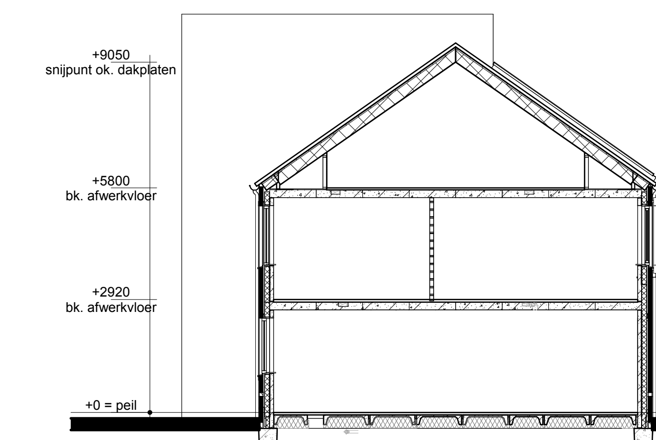
Doorsnede A2-A2
