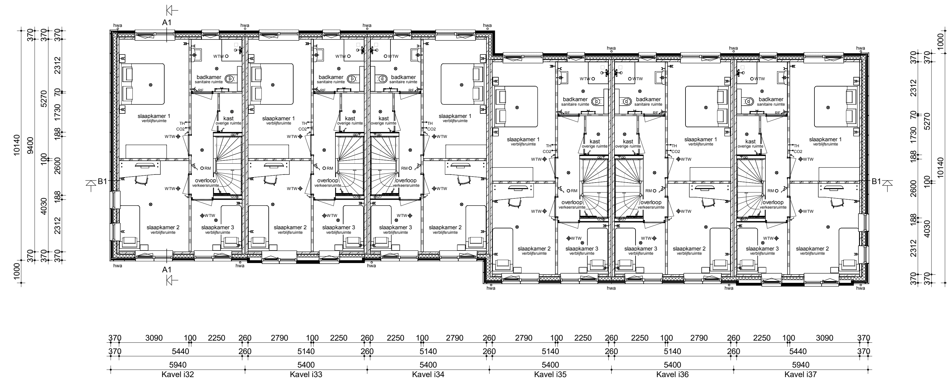
Verdieping
