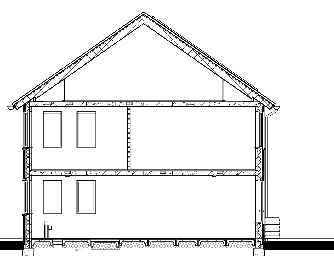
Doorsnede A1-A1
