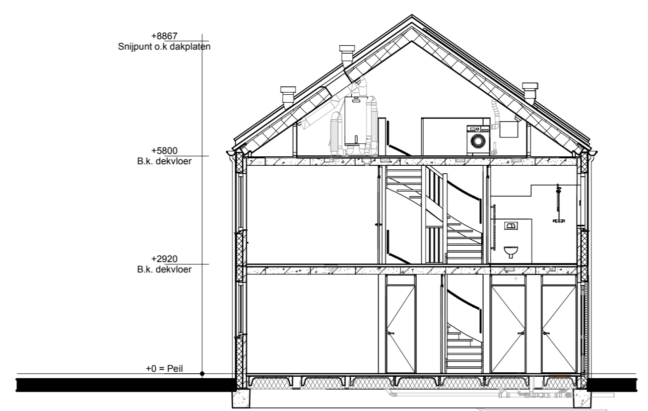
Doorsnede A1-A1
