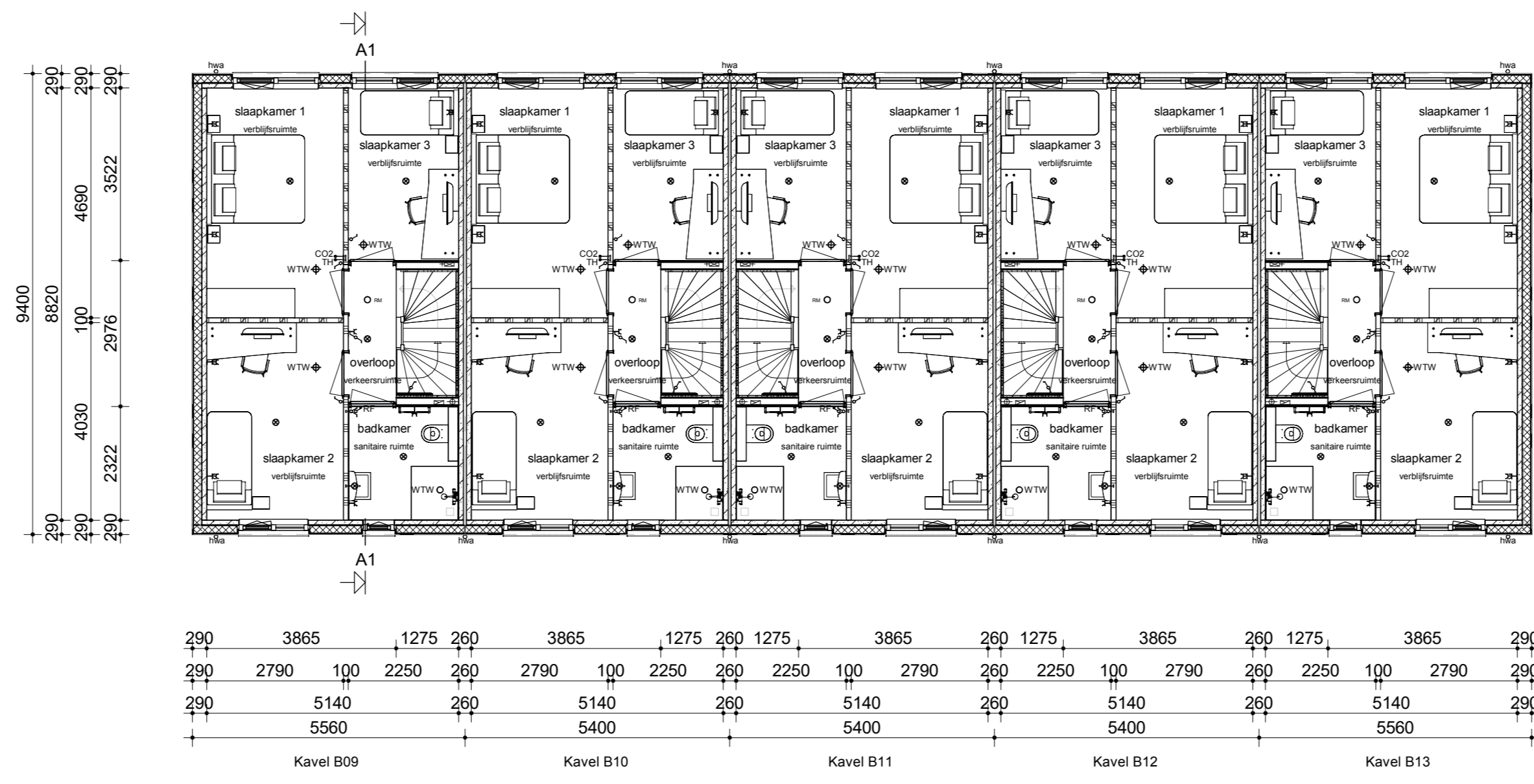
Verdieping
