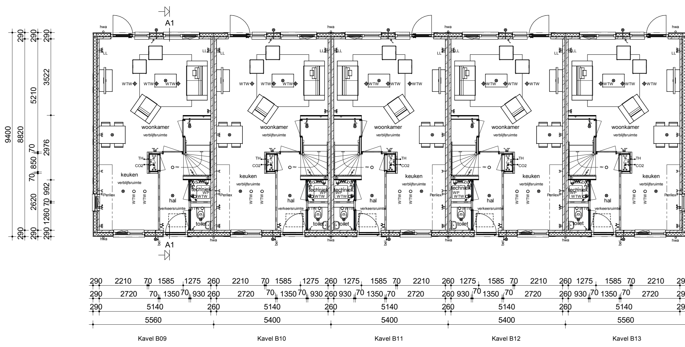
Begane grond
