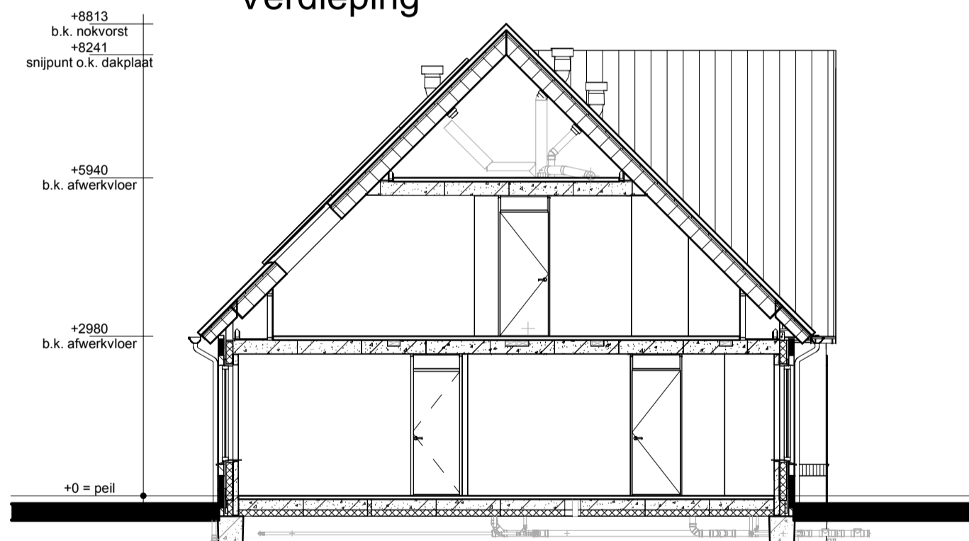
Doorsnede A1-A1
