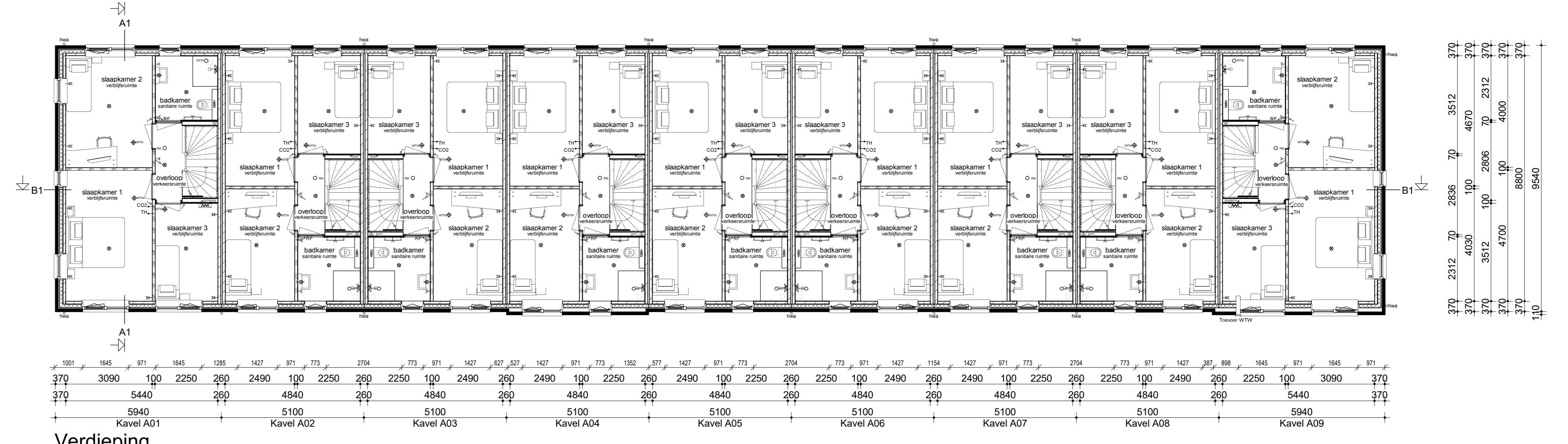
Verdieping
