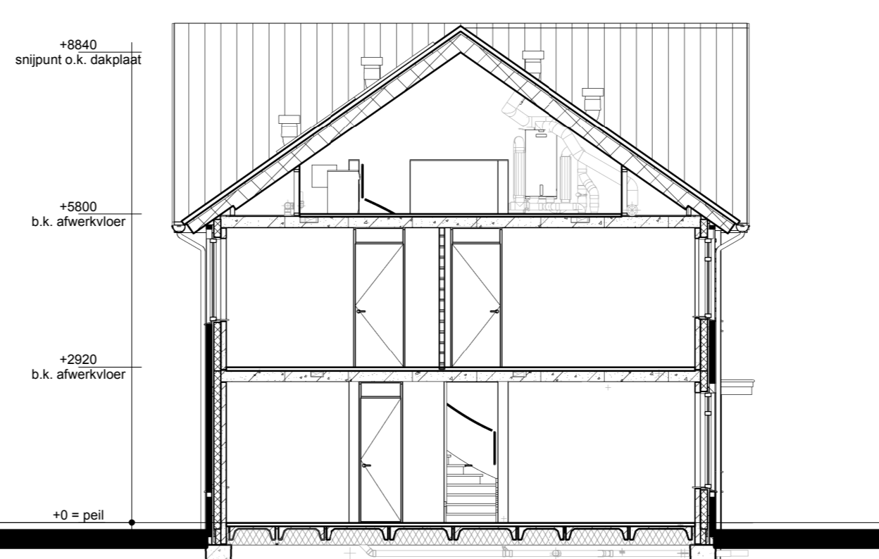
Doorsnede A1-A1
