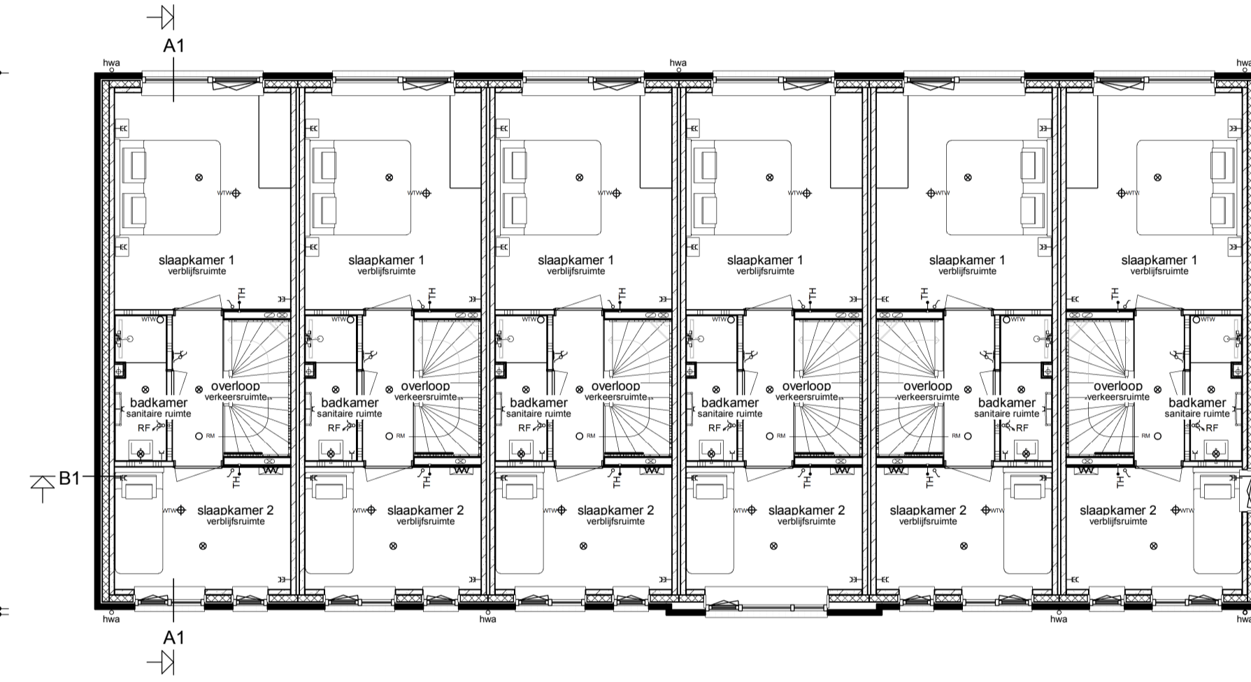
Verdieping
