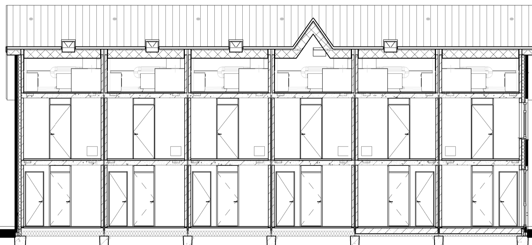
Doorsnede B1-B1
