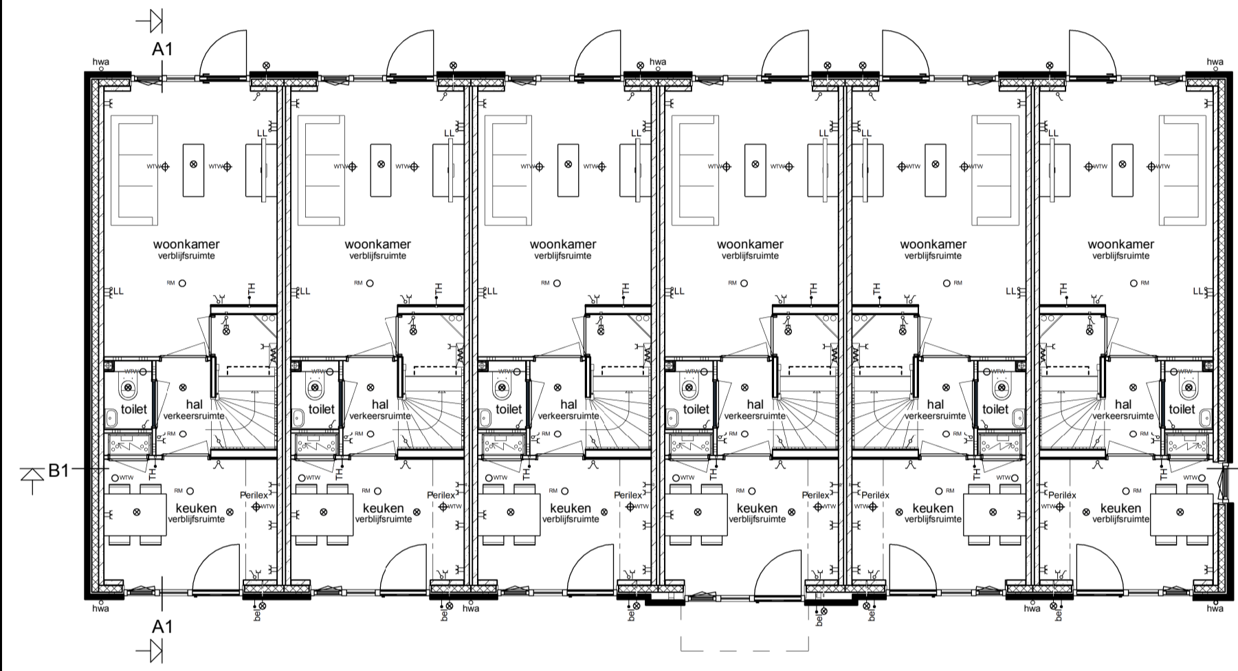
Begane grond
