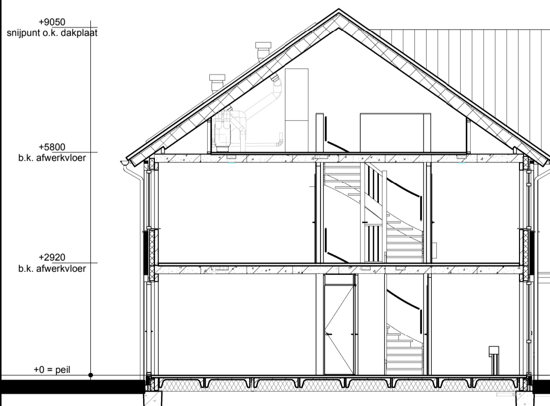
Doorsnede A1-A1
