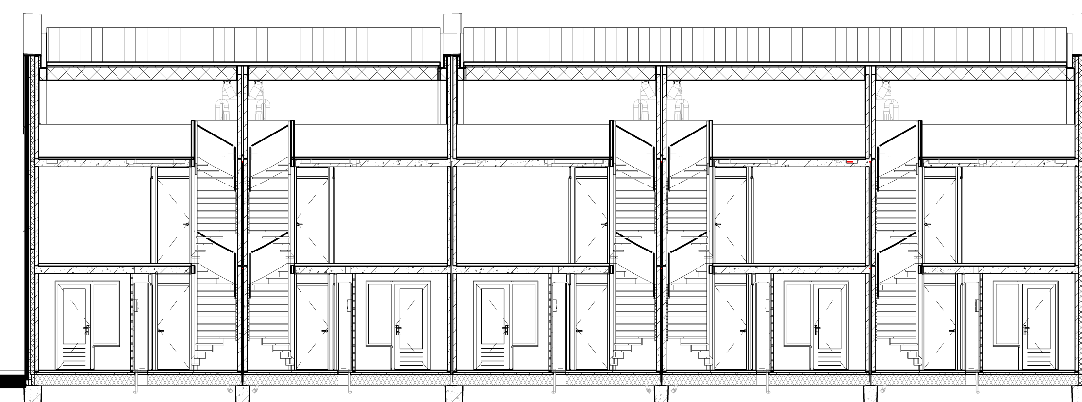
Doorsnede B2-B2
