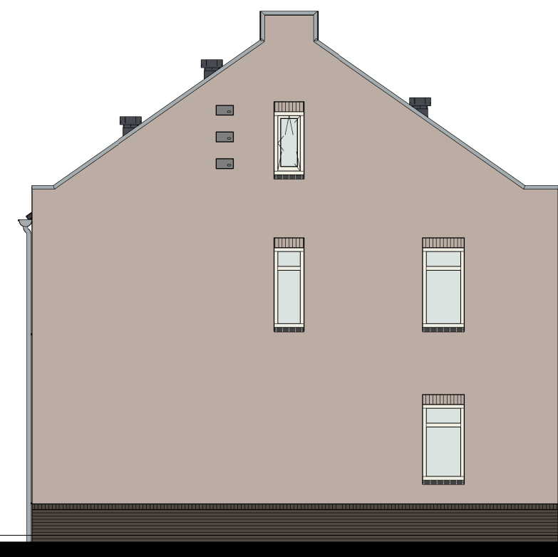
Linker zijgevel
