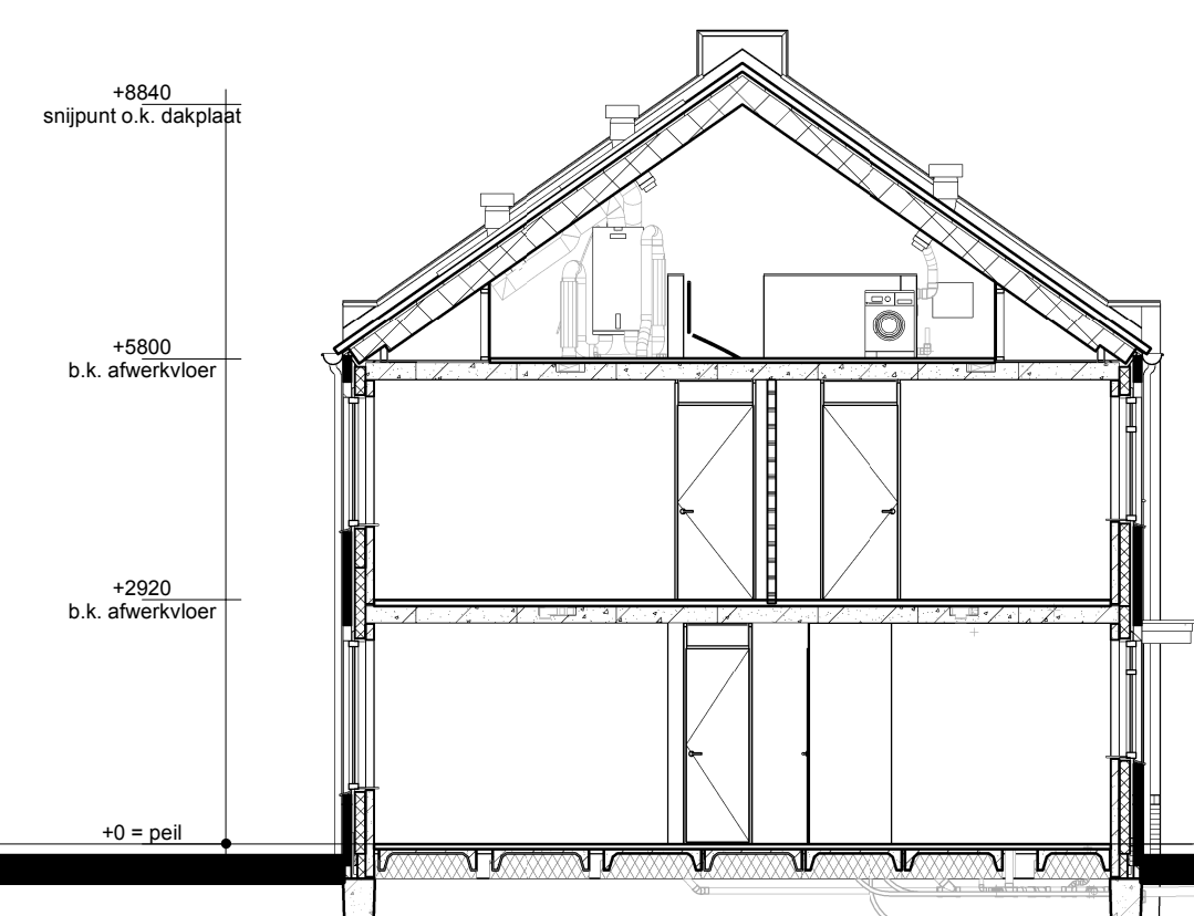
Doorsnede A2-A2
