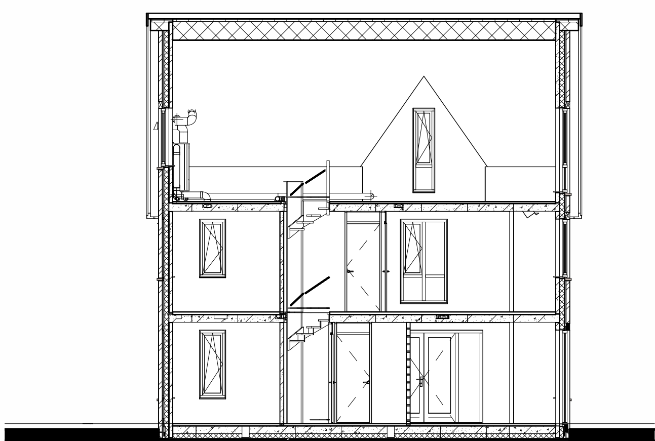
Doorsnede B1-B1
