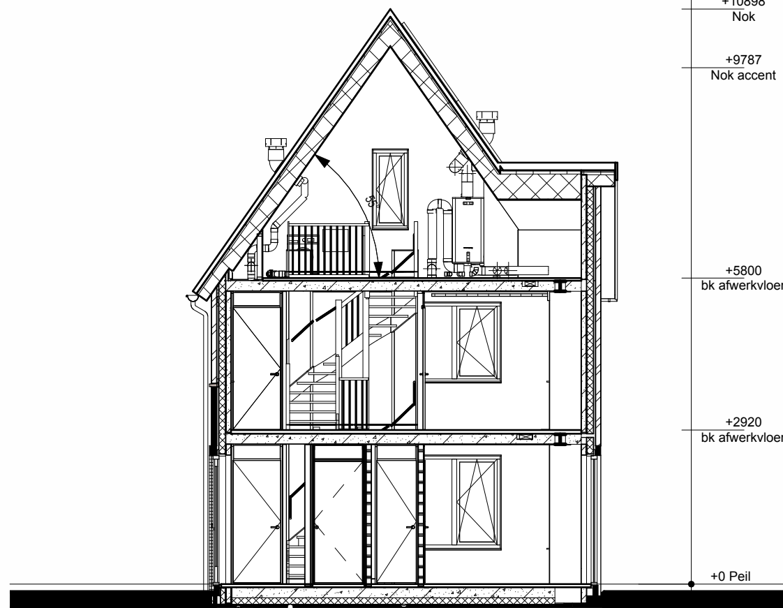
Doorsnede A1-A1
