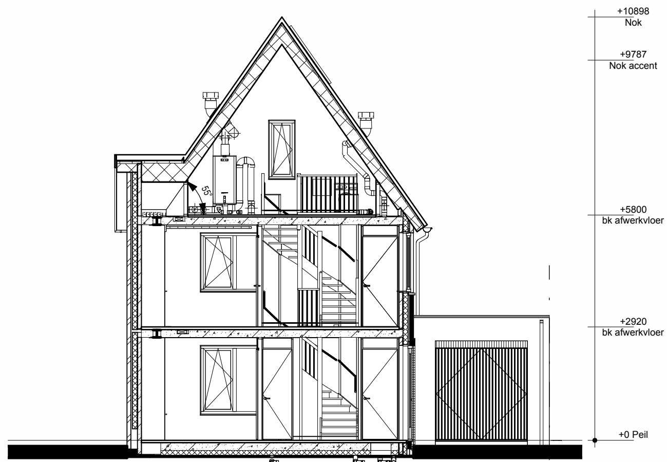
Doorsnede A1-A1
