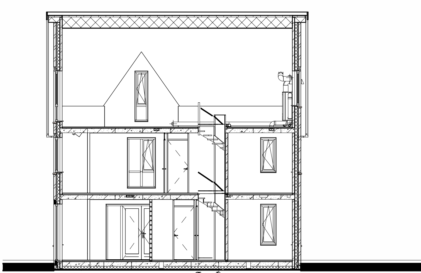
Doorsnede B1-B1
