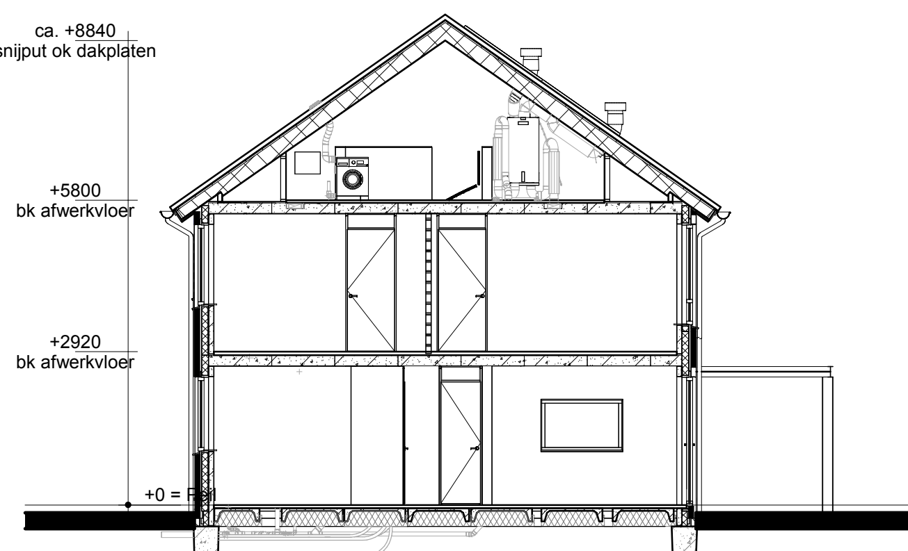
Doorsnede A1-A1
