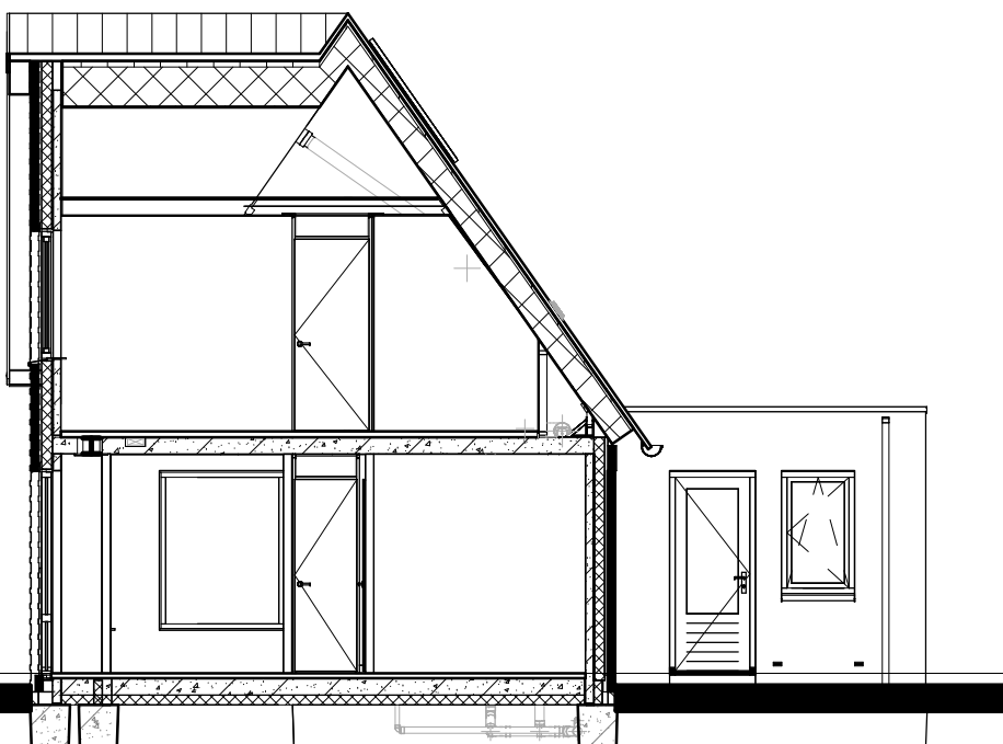
Doorsnede B1-B1
