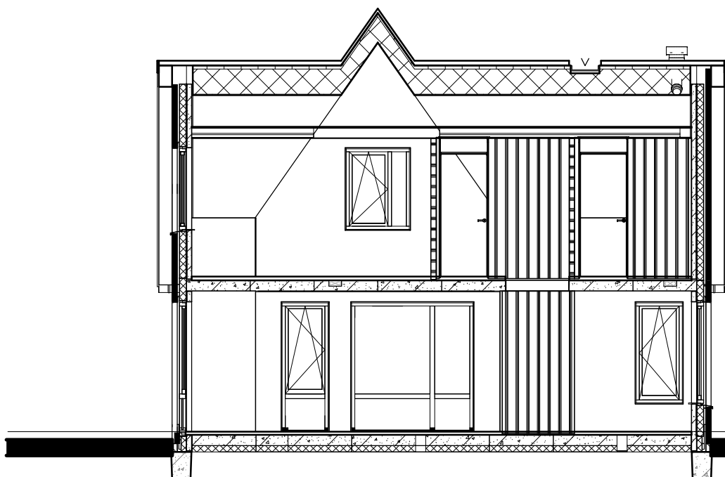
Doorsnede A1-A1
