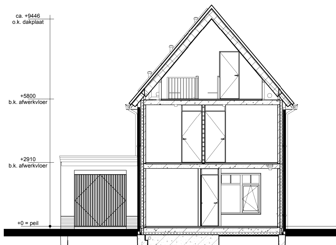
Doorsnede AA
