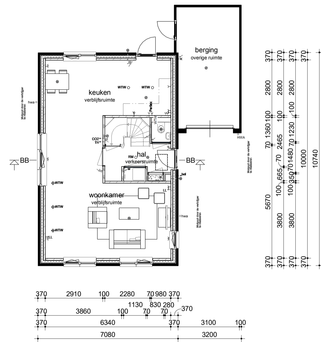
Begane grond
