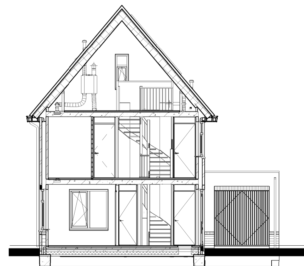
Doorsnede BB
