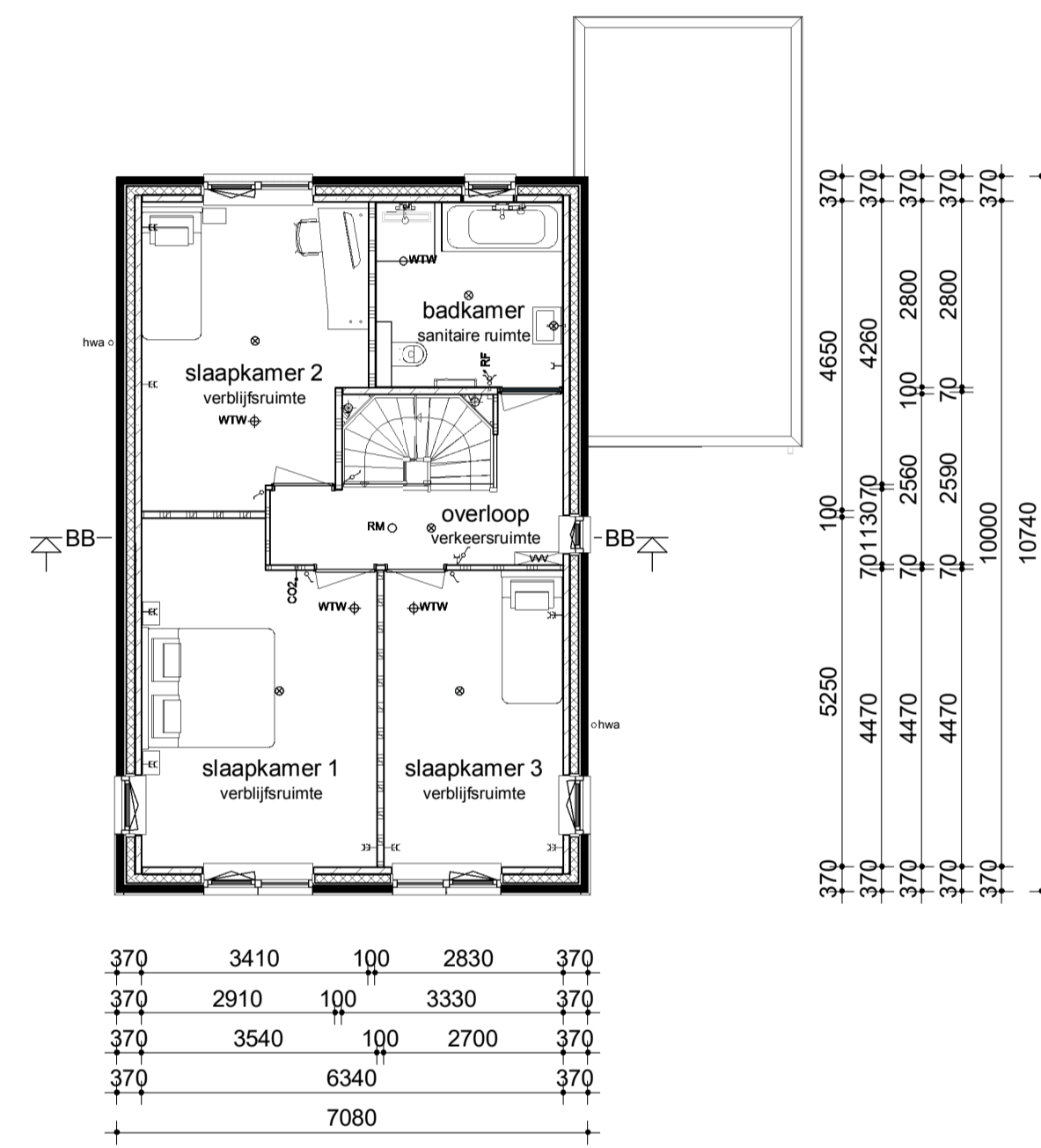
Verdieping
