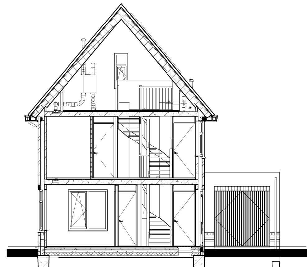
Doorsnede BB
