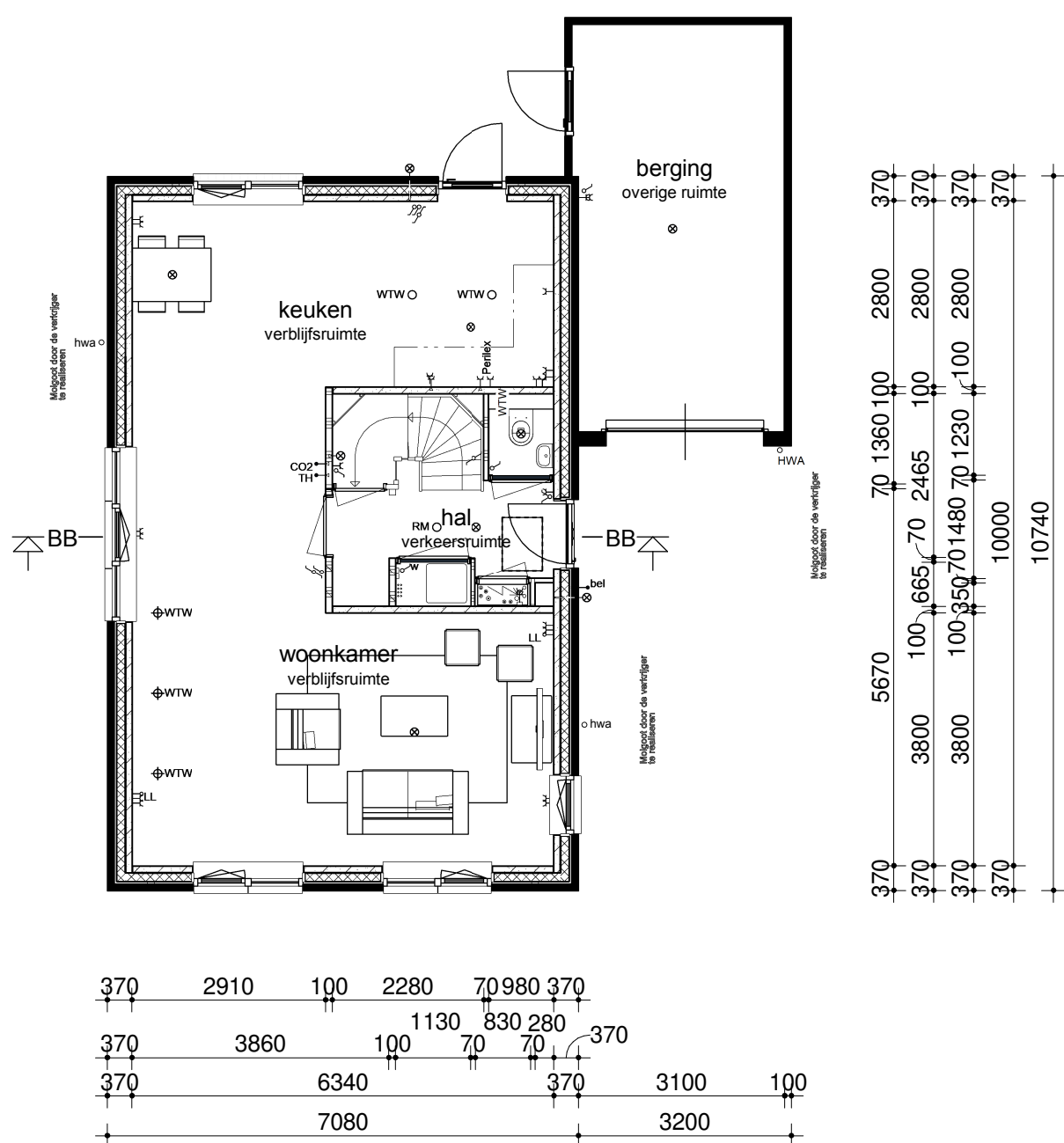
Begane grond
