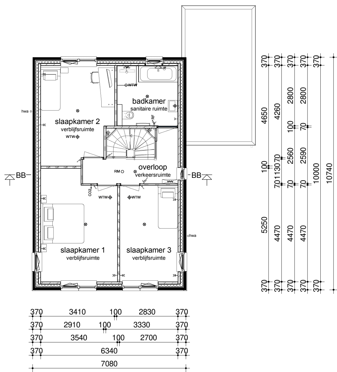
Verdieping
