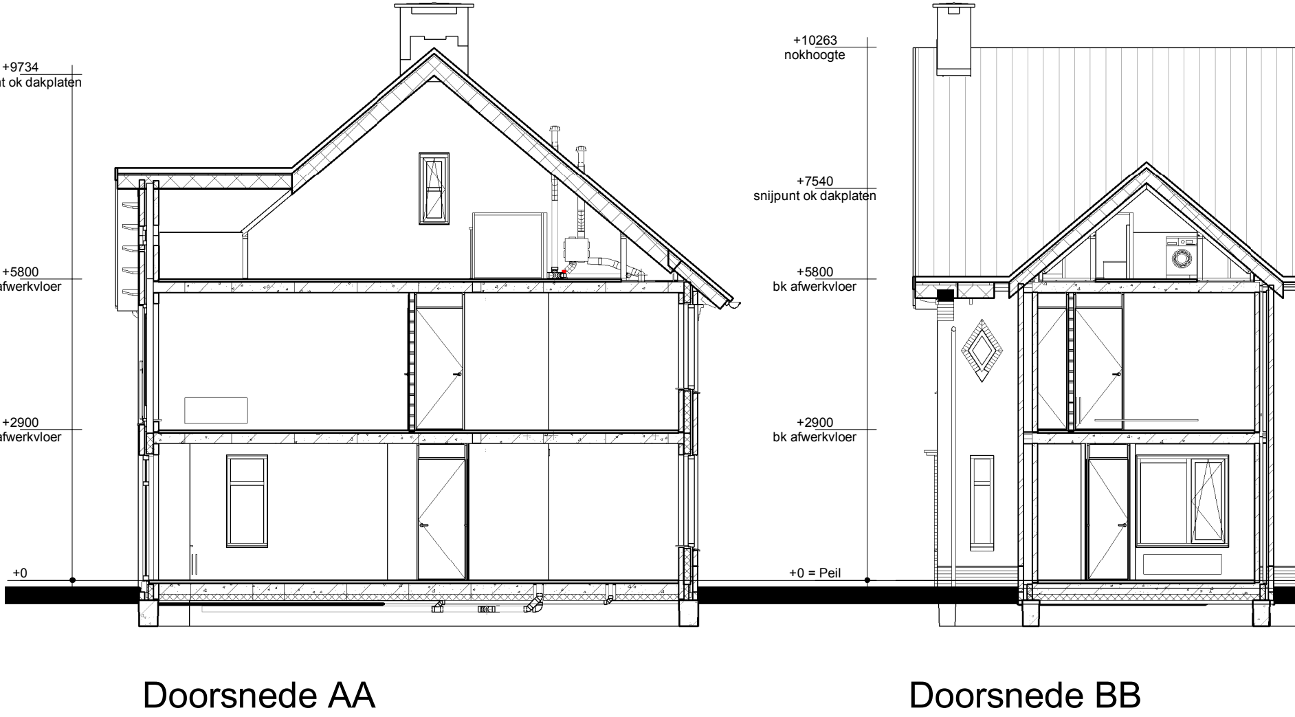
Doorsnede AA
