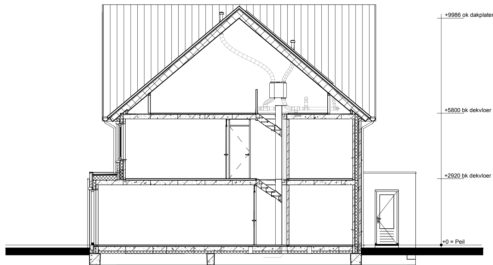
Doorsnede AA
