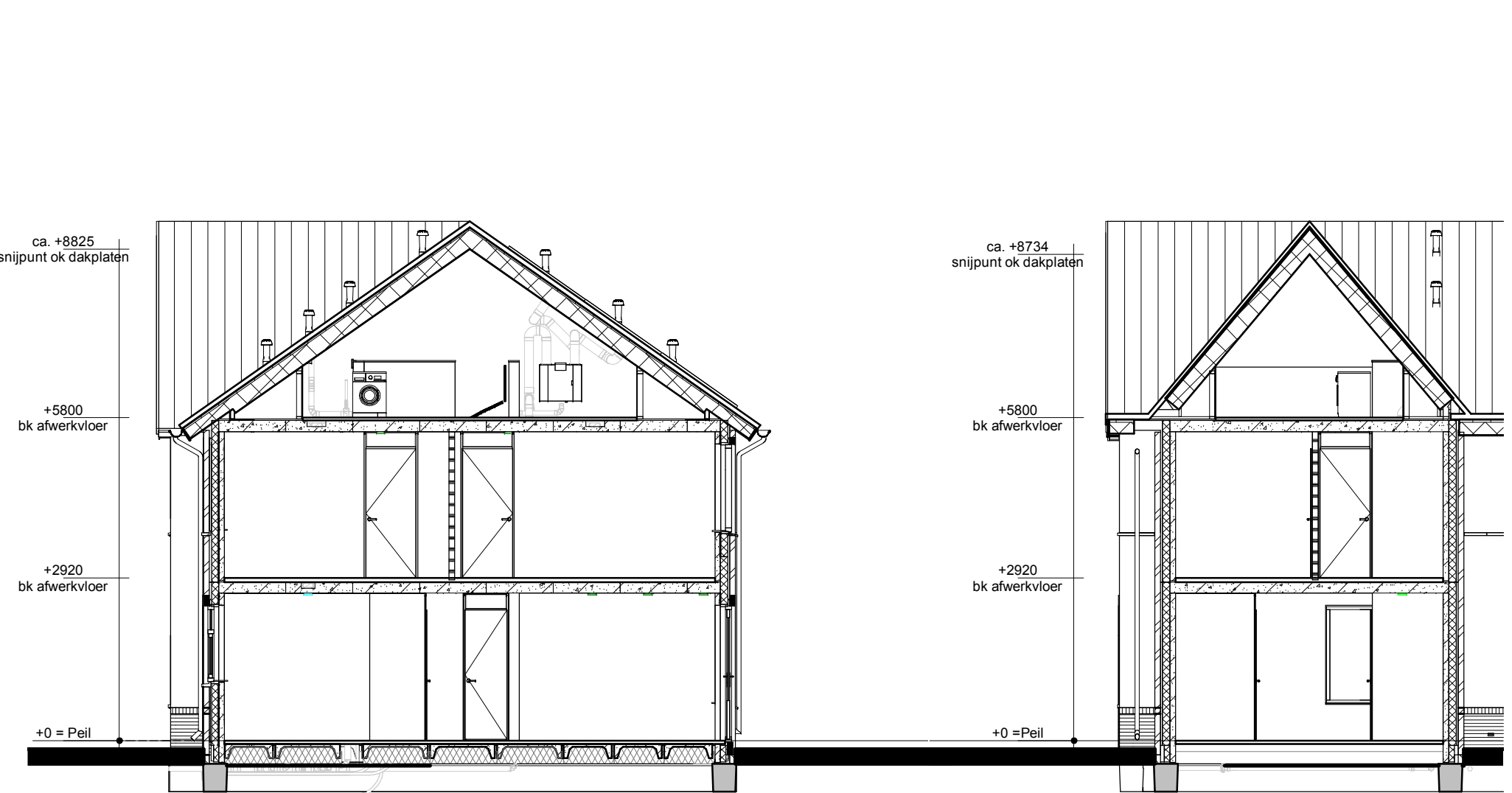
Doorsnede A1-A1
