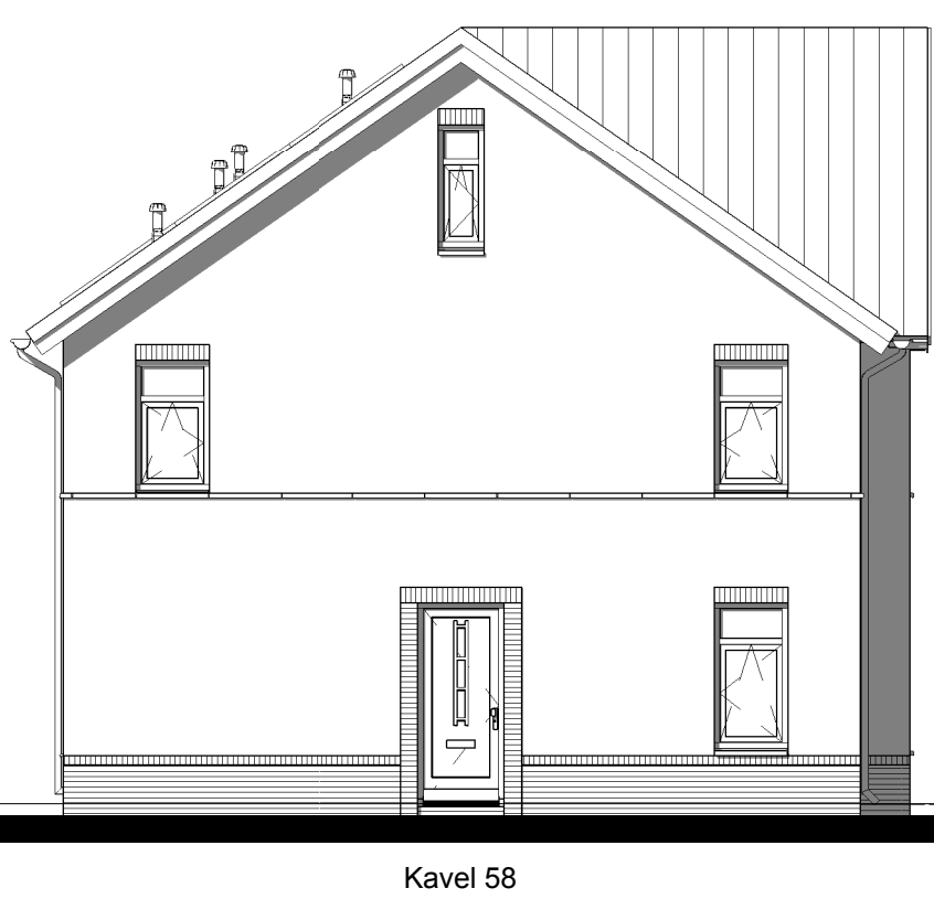
Linker zijgevel
