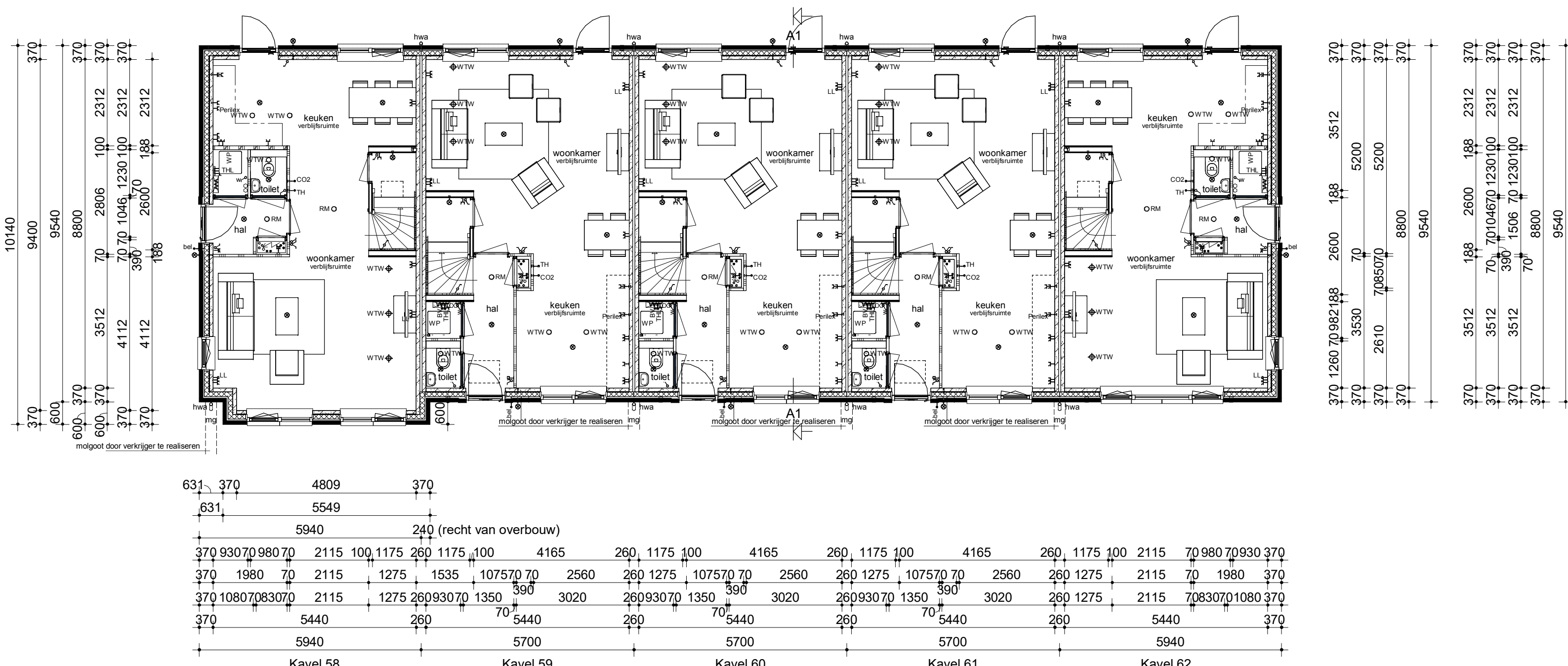
Begane grond
