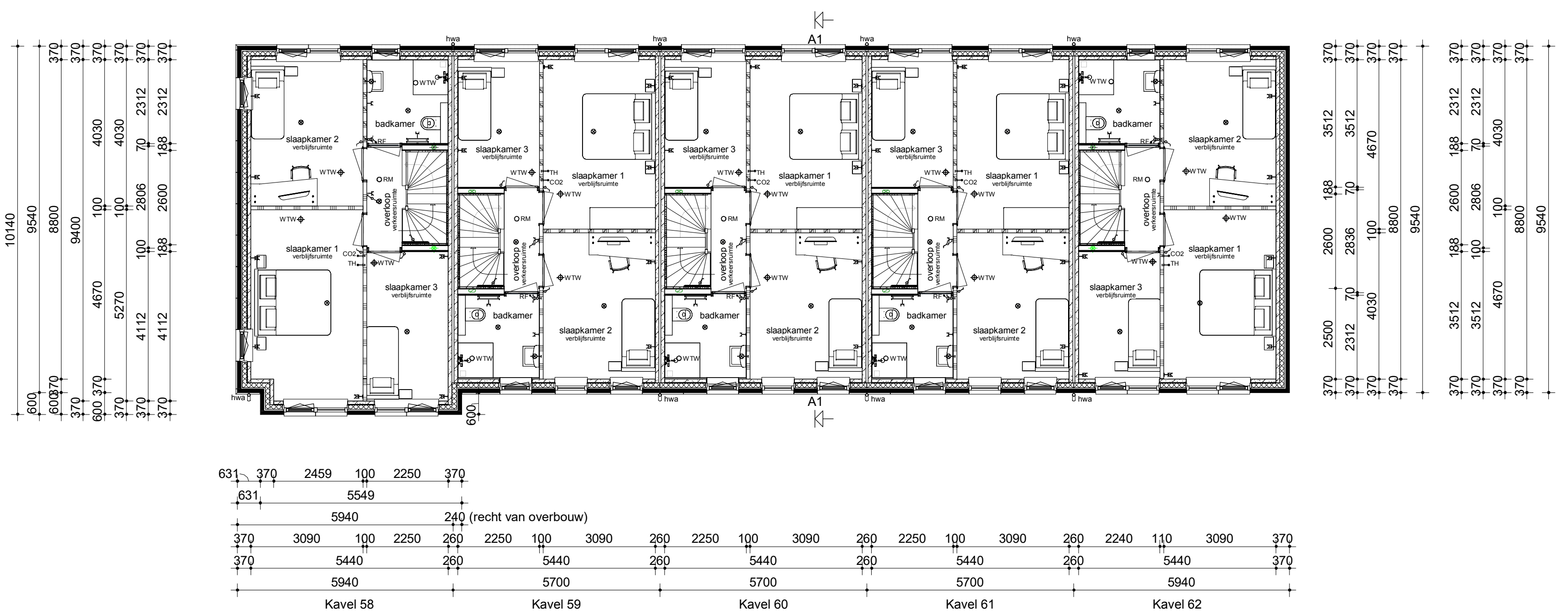
Verdieping
