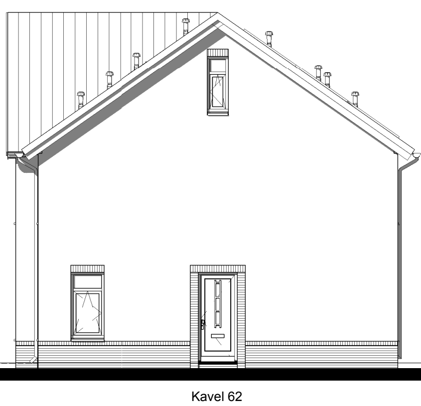
Rechter zijgevel
