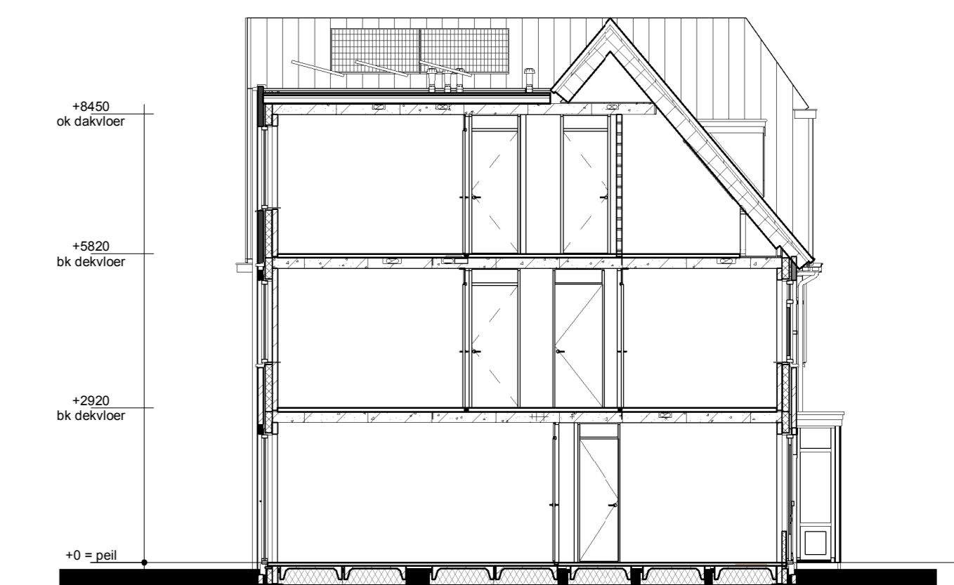
Doorsnede AA
