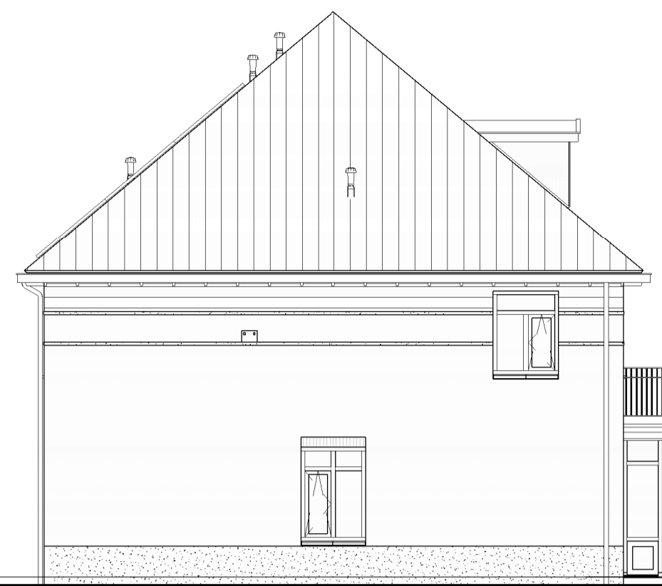
Linker zijgevel
