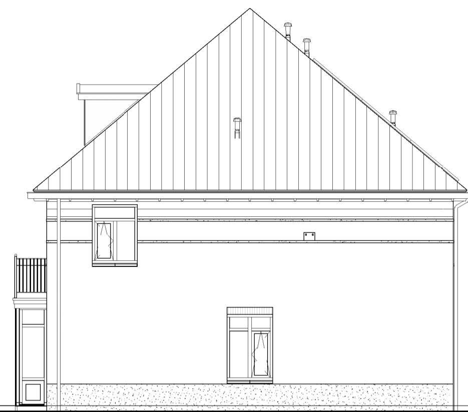
Rechter zijgevel
