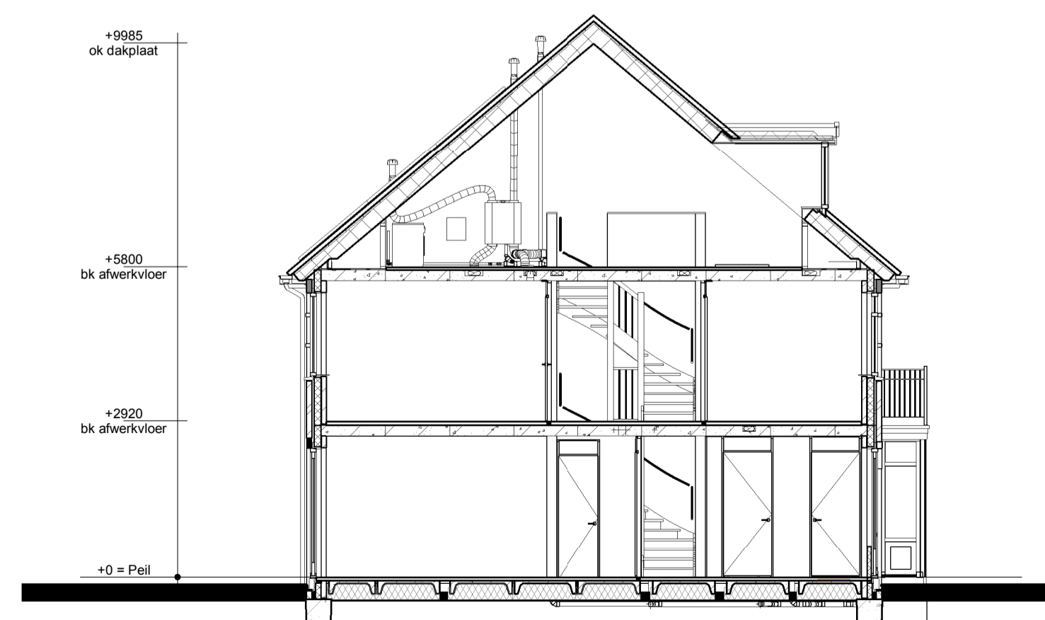
Doorsnede AA
