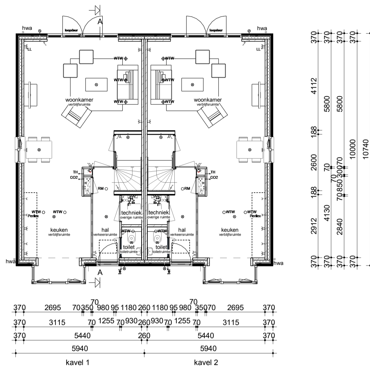
Begane grond
