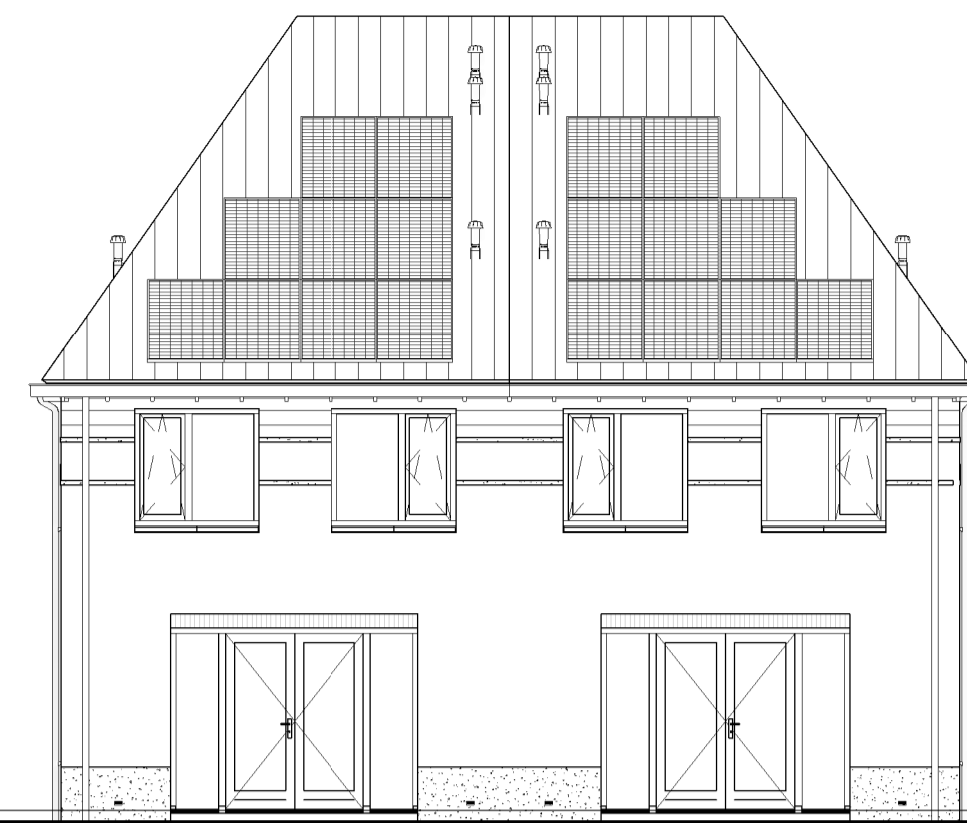
Achtergevel
