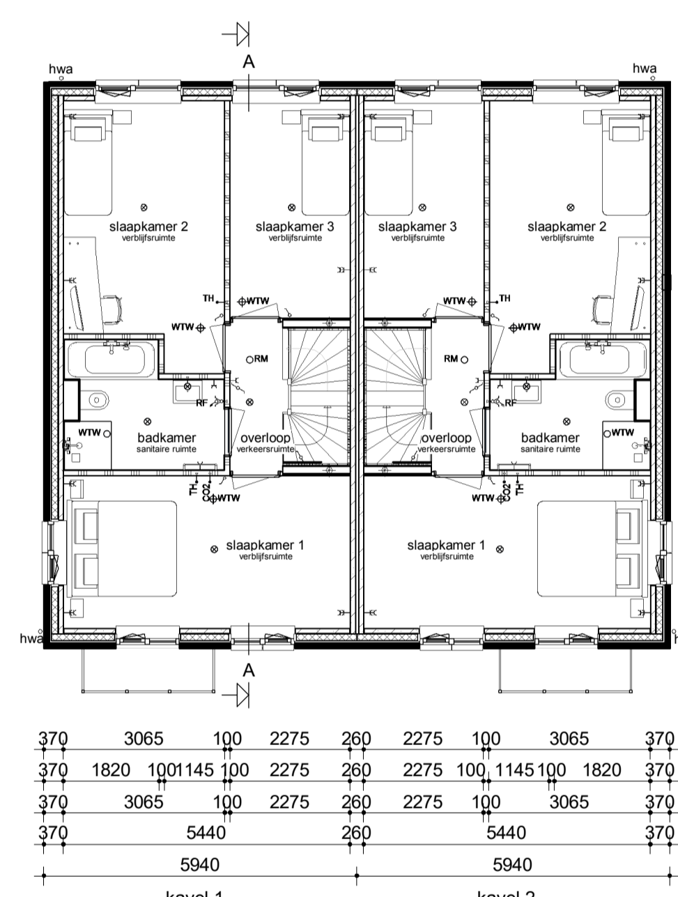
Verdieping
