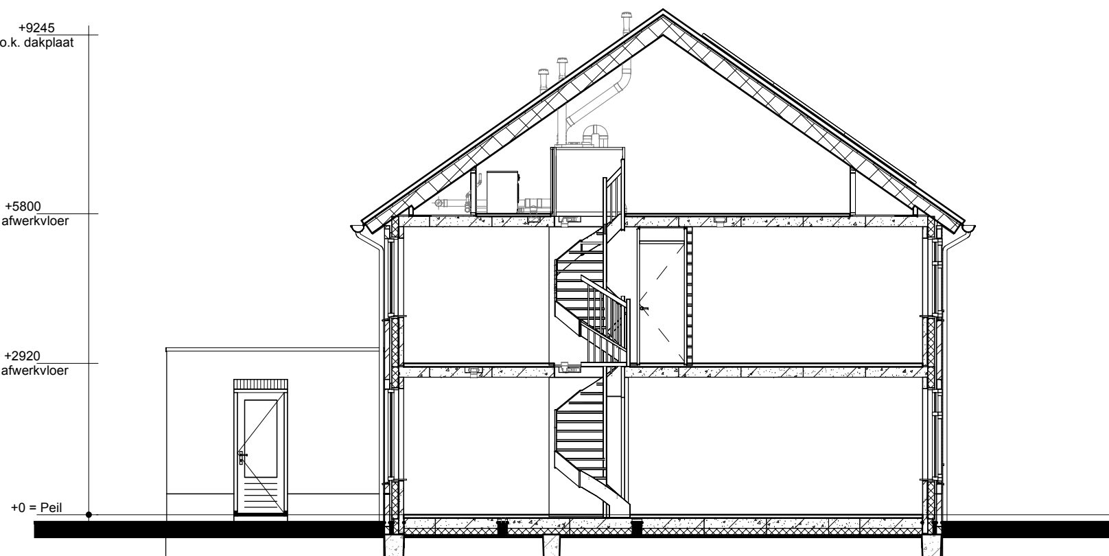
Doorsnede A1-A1
