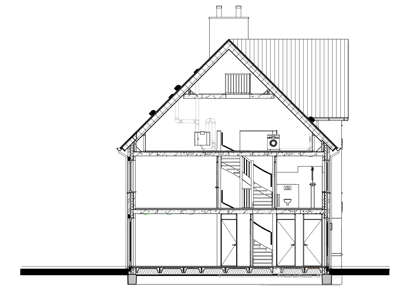
Doorsnede A4-A4
