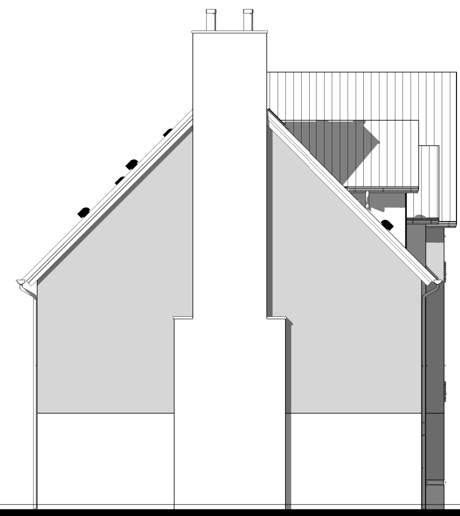
Linker zijgevel
