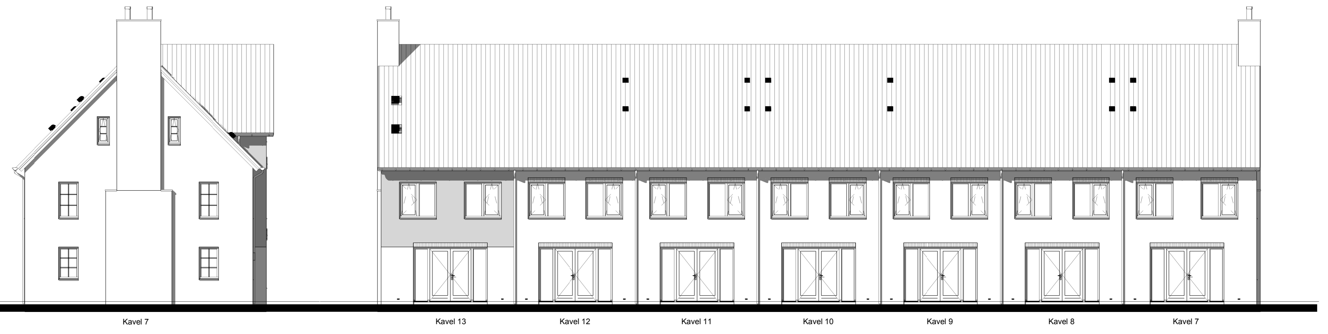
Linker zijgevel
