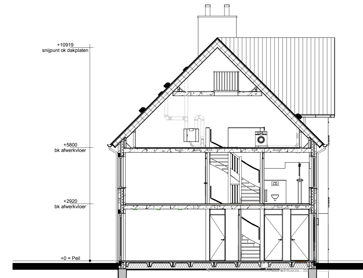
Doorsnede A2-A2
