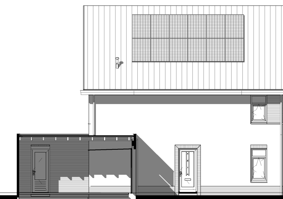
Linker zijgevel
