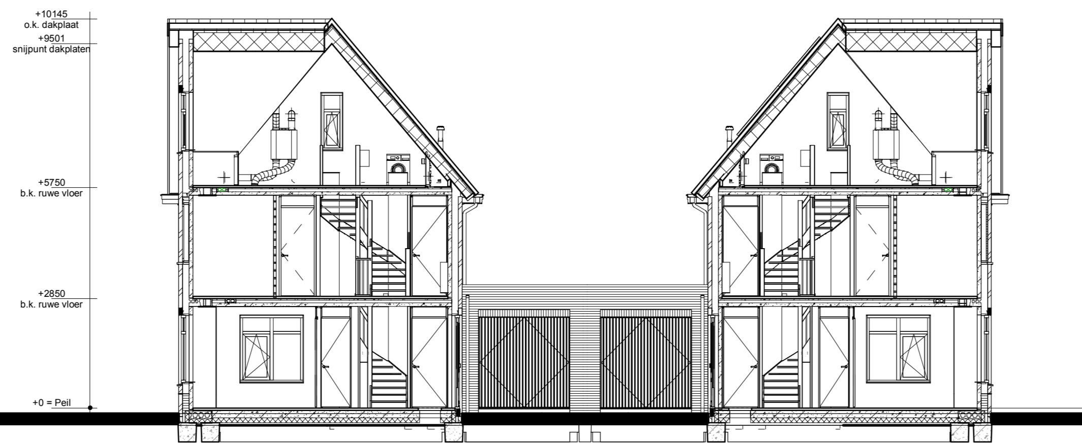
Doorsnede BB
