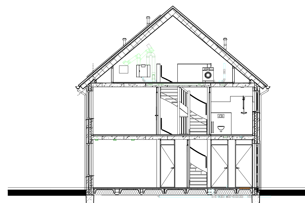
Doorsnede AA
