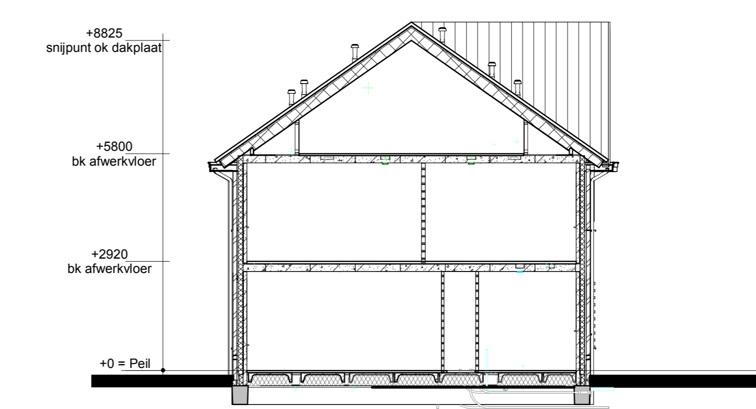
Doorsnede A3
