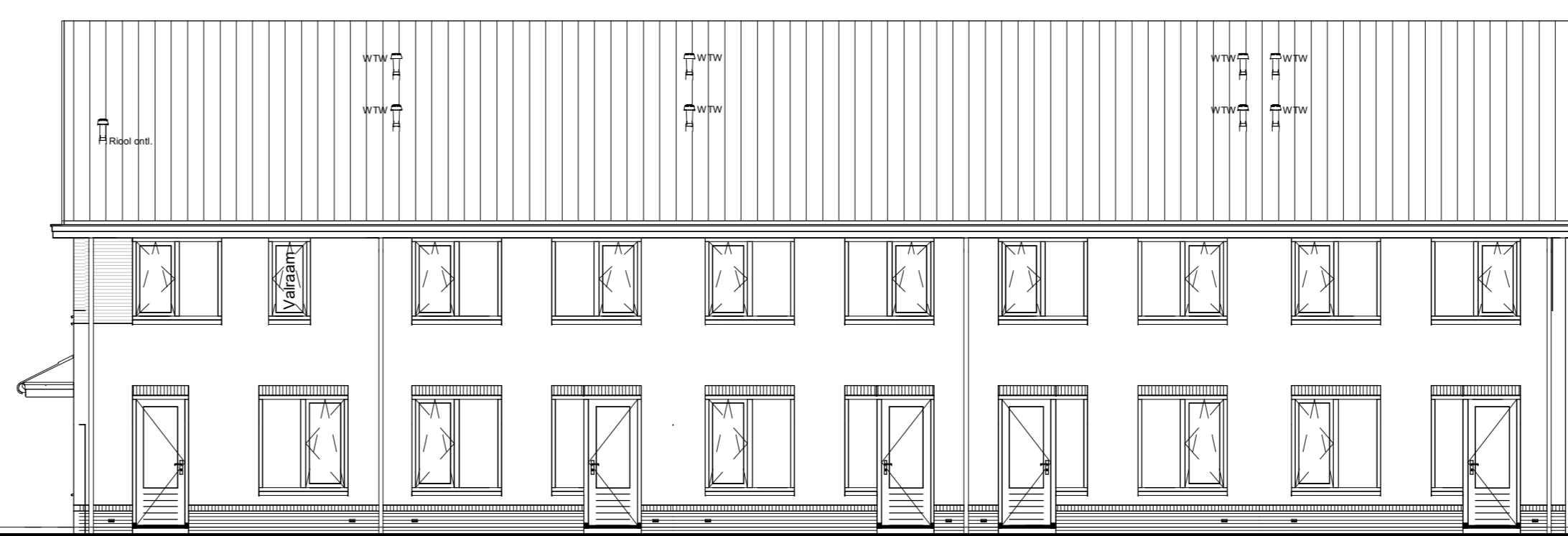
Achtergevel
