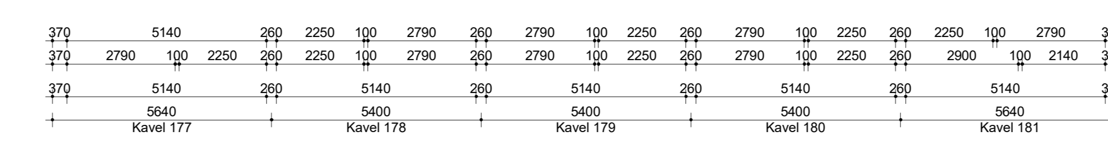
Verdieping
