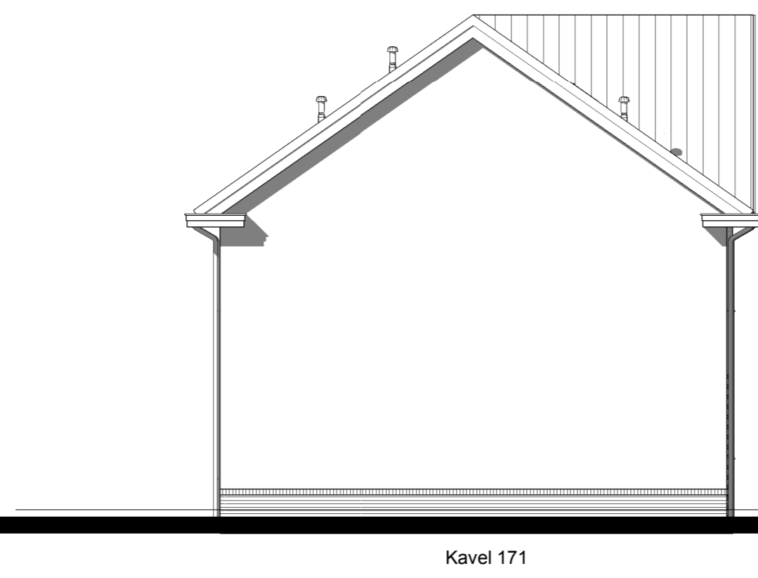
Linker zijgevel
