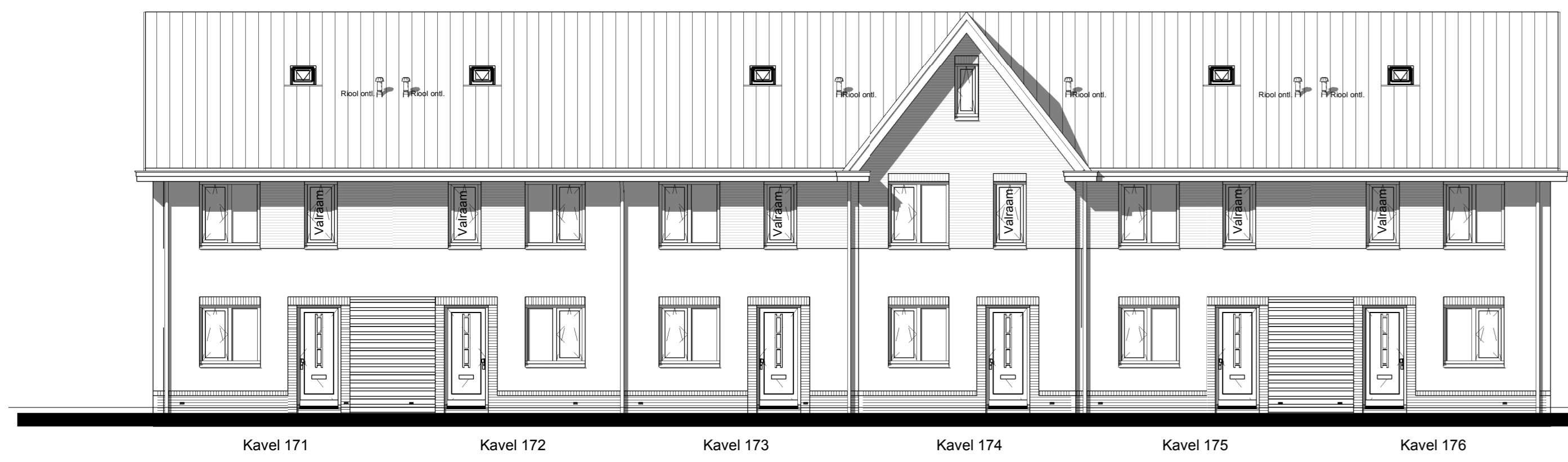
Voorgevel
