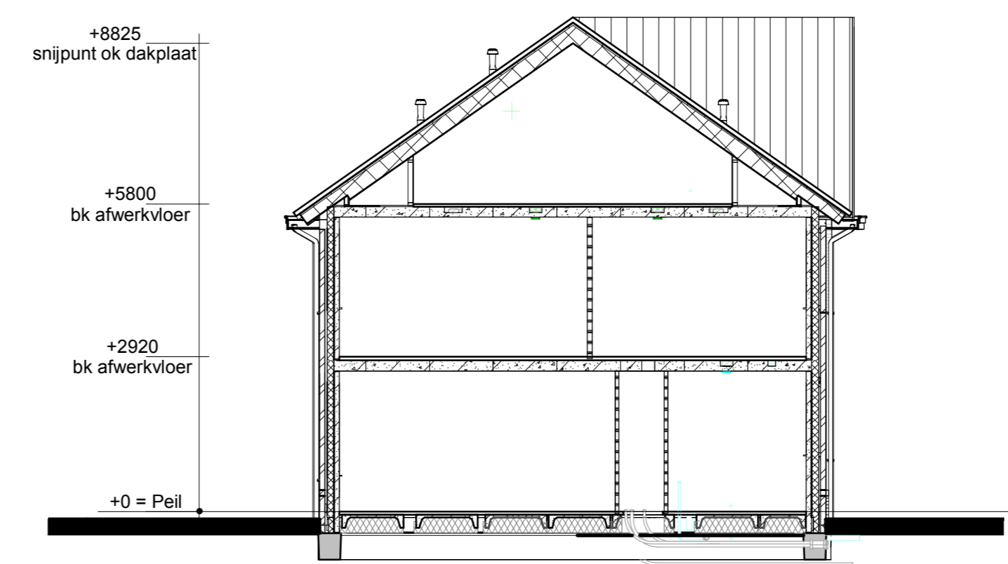
Doorsnede AA
