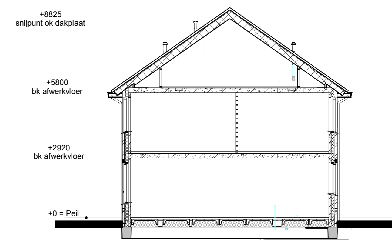
Doorsnede A2
