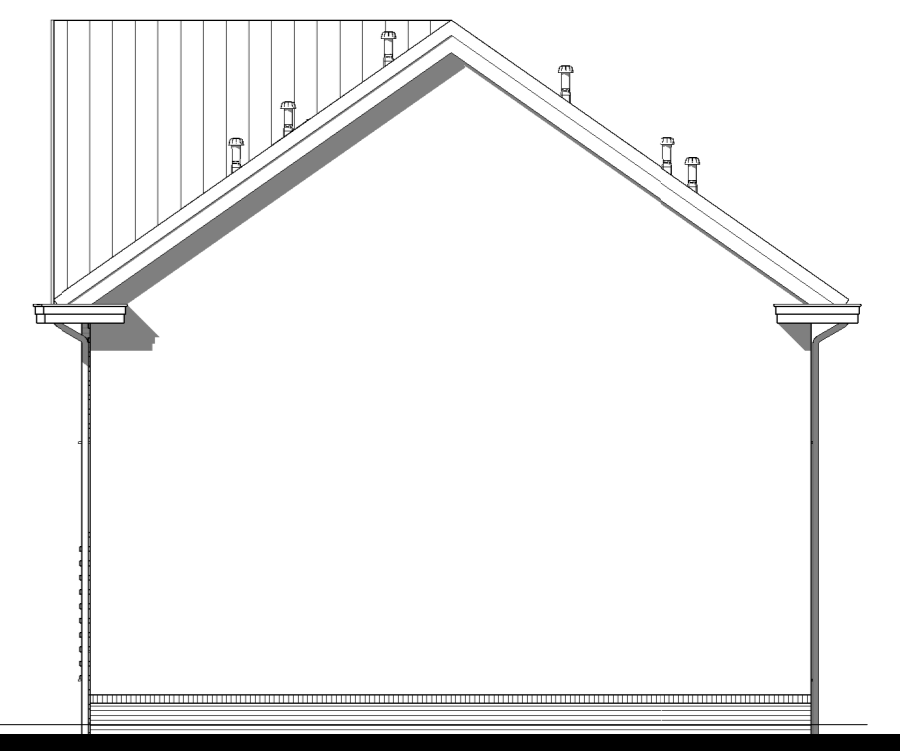
Rechter zijgevel
