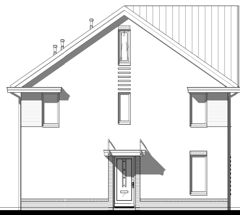
Linker zijgevel
