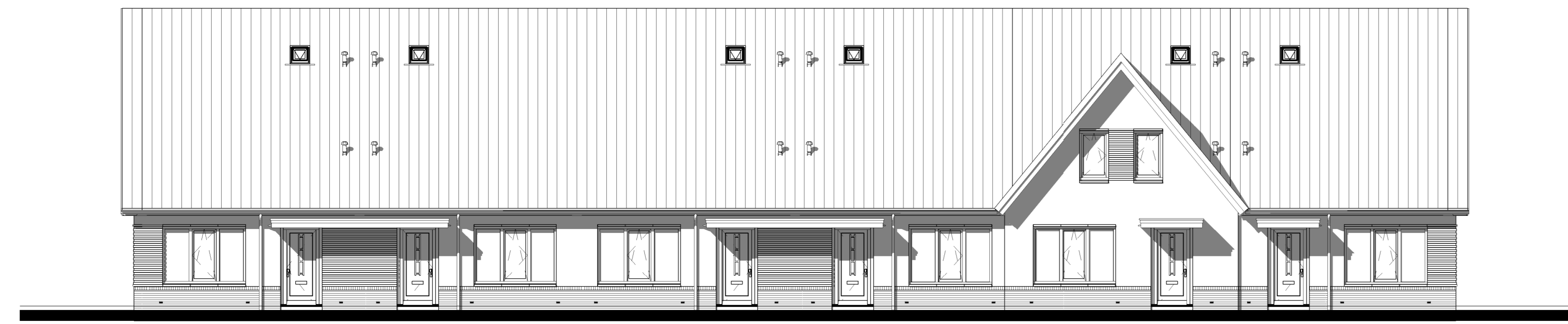
Voorgevel
