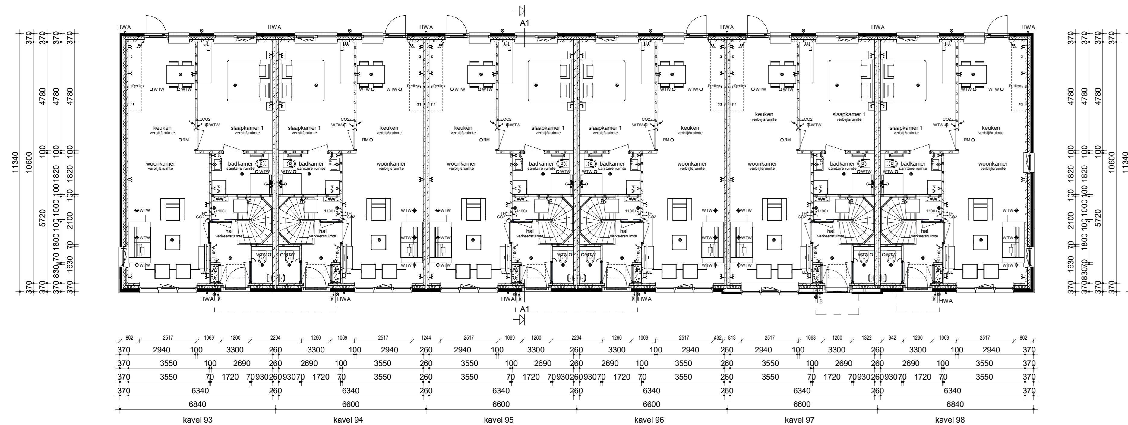
Begane grond
