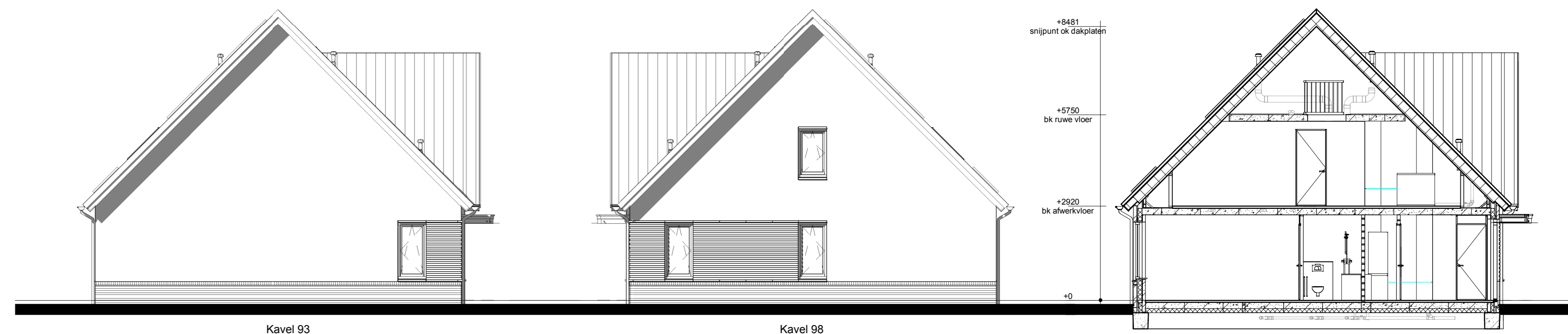
Linker zijgevel
