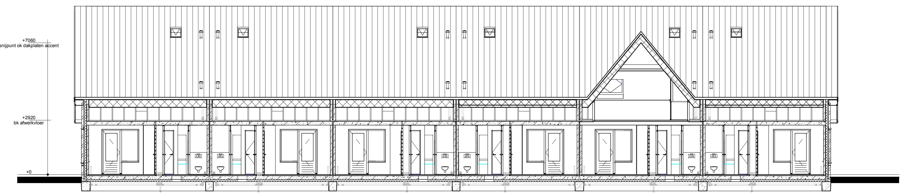
Doorsnede BB
