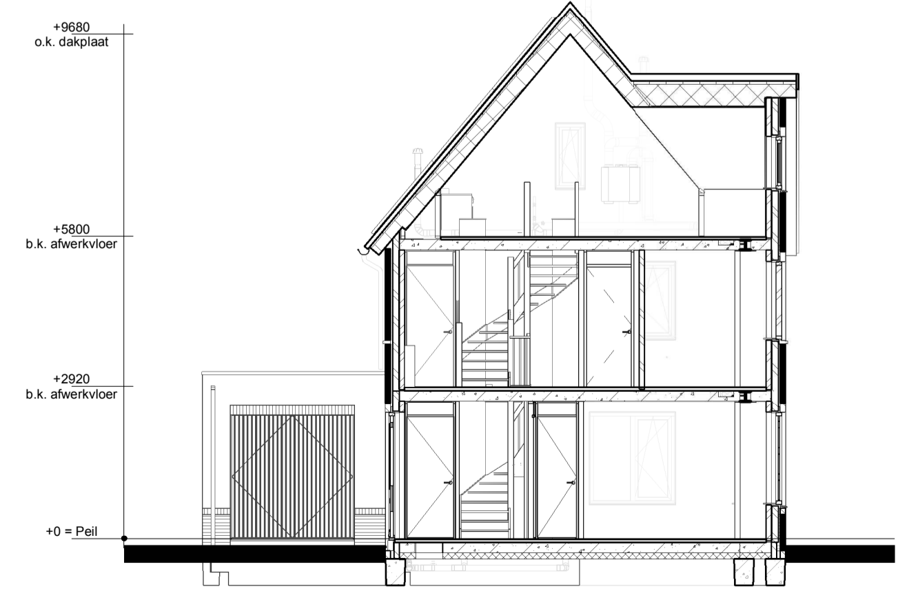
Doorsnede A-A
