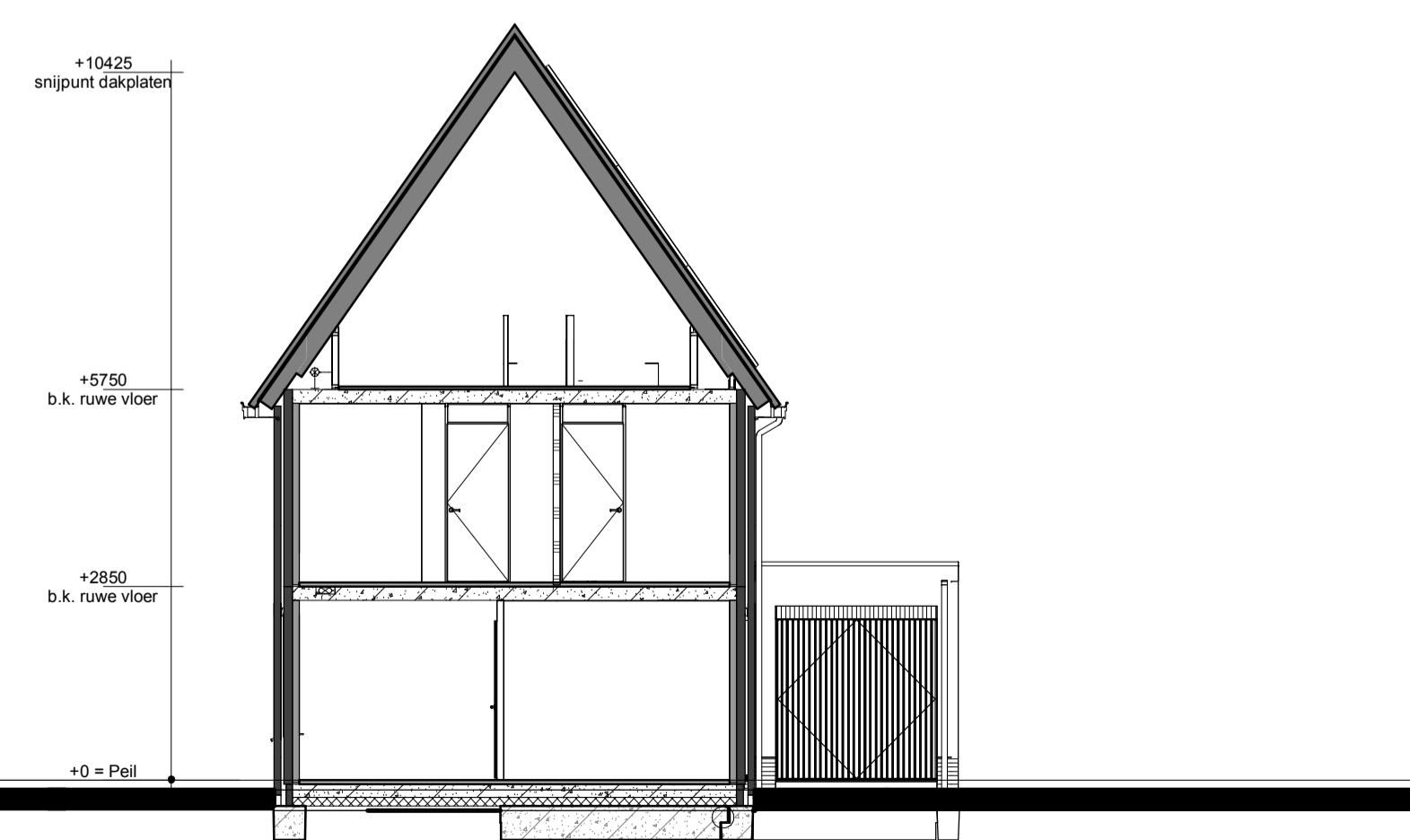
Doorsnede BB
