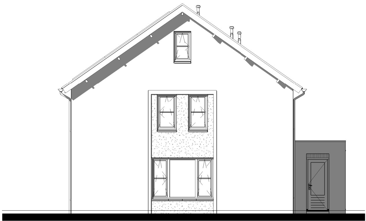
Rechter zijgevel
