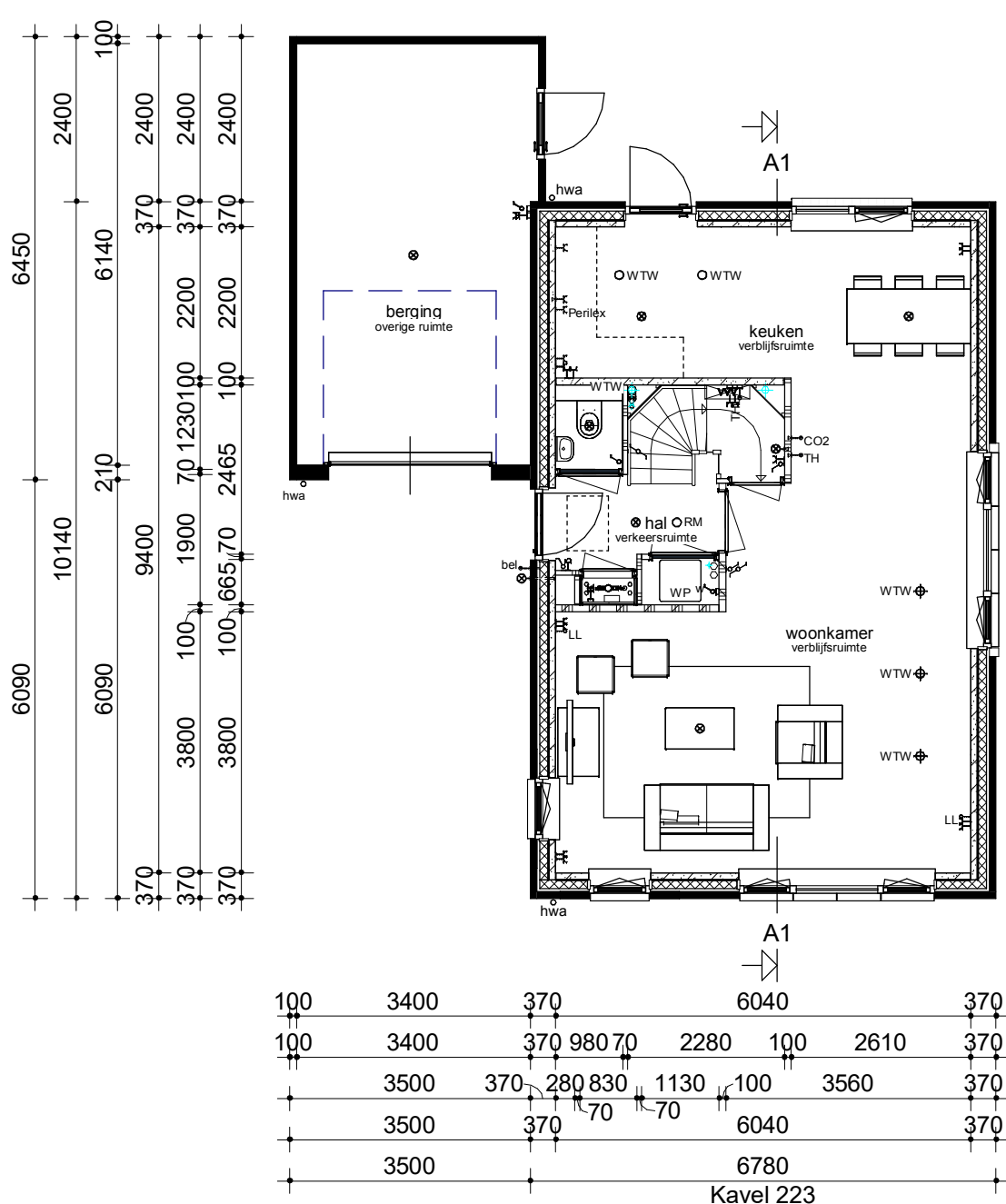
Begane grond
