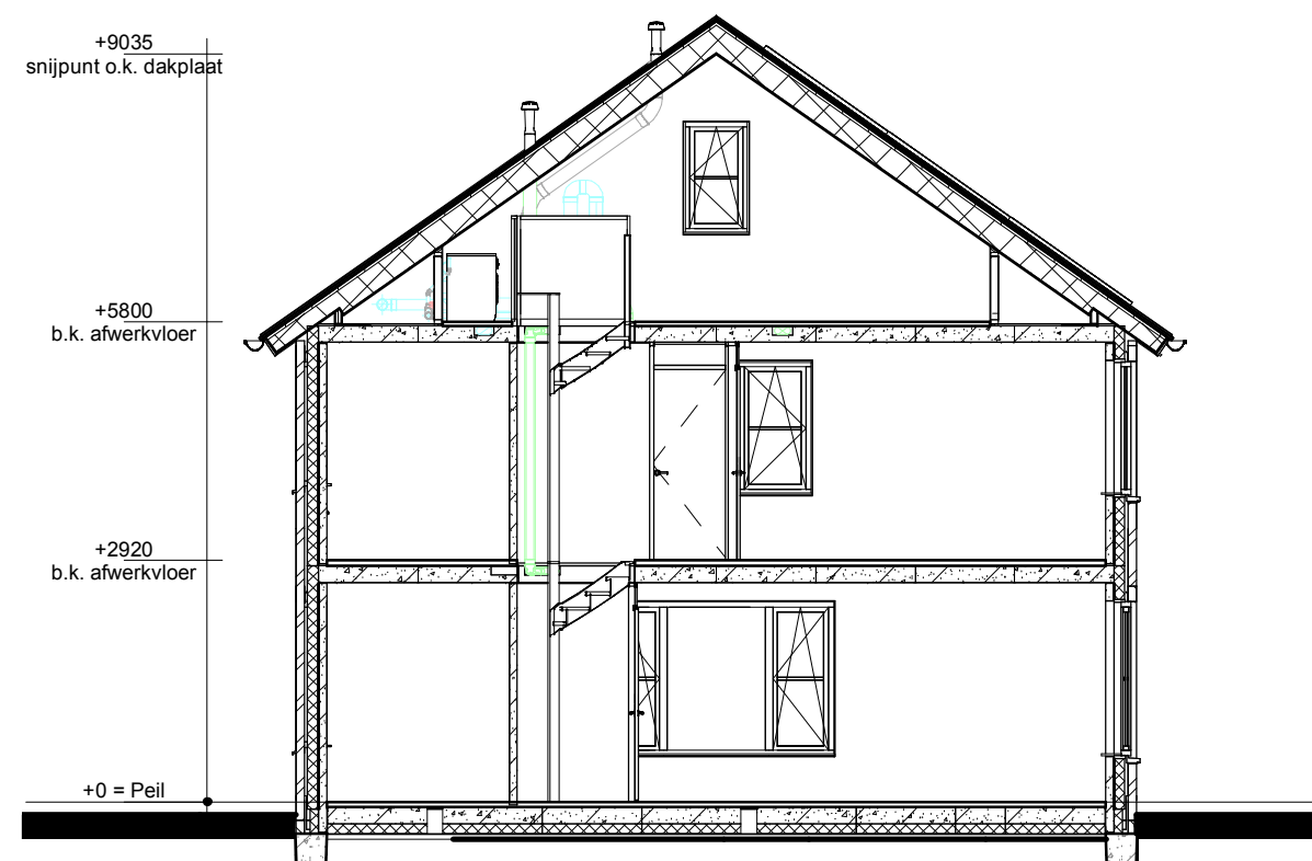
Doorsnede A1
