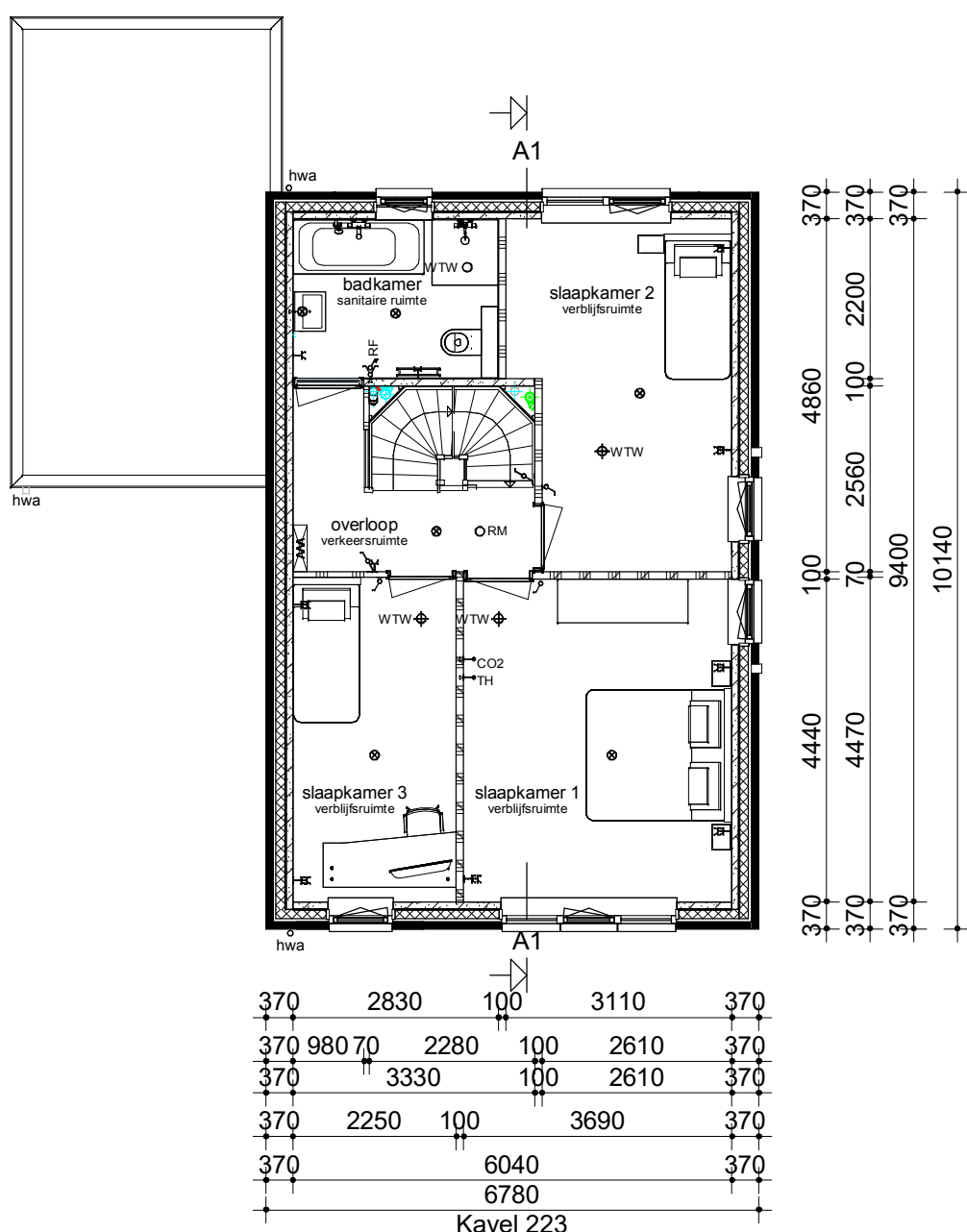
Verdieping
