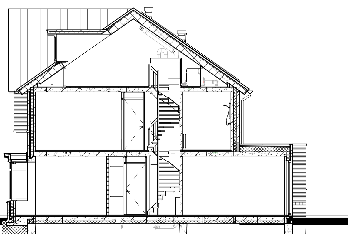
Doorsnede A4
