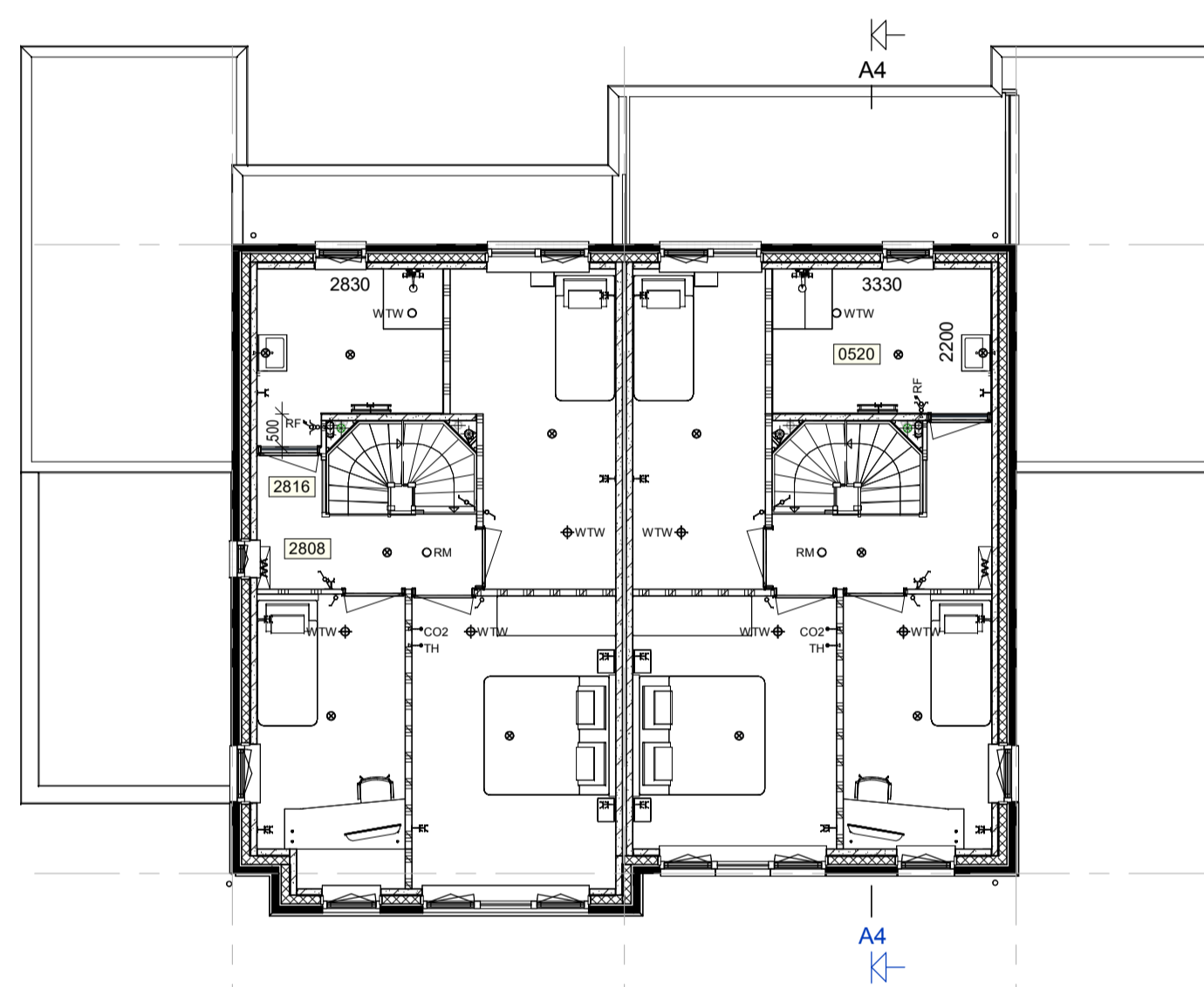
Verdieping
