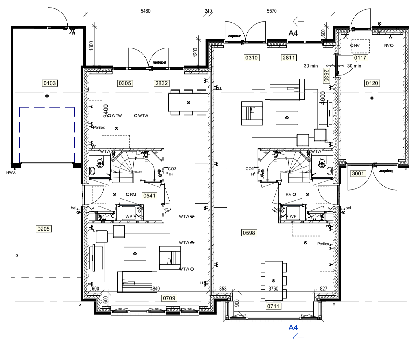
Begane grond
