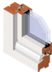
Hardhouten buitengevelkozijn (draaikiep en triple glas is optioneel)
