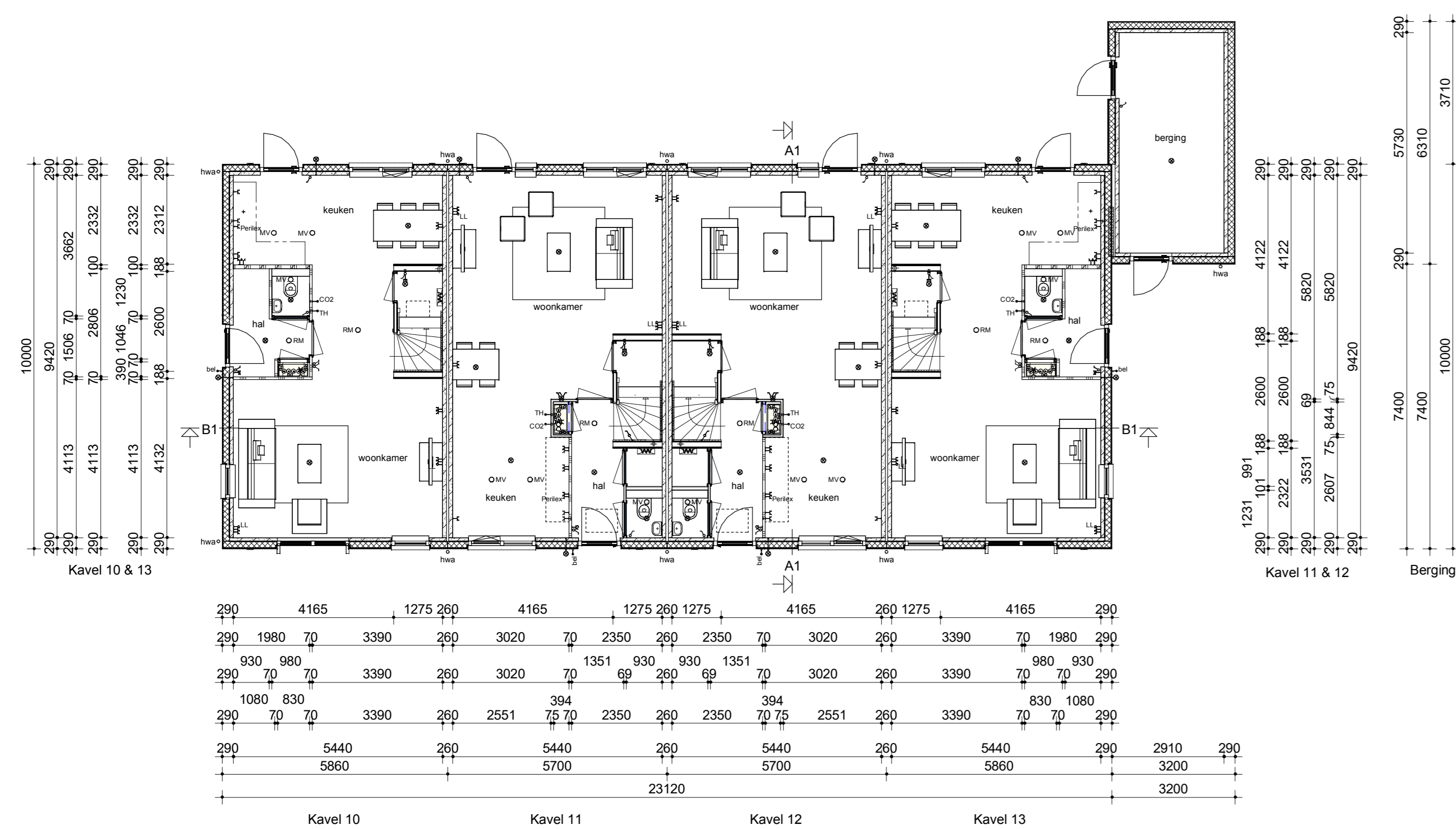
Begane grond
