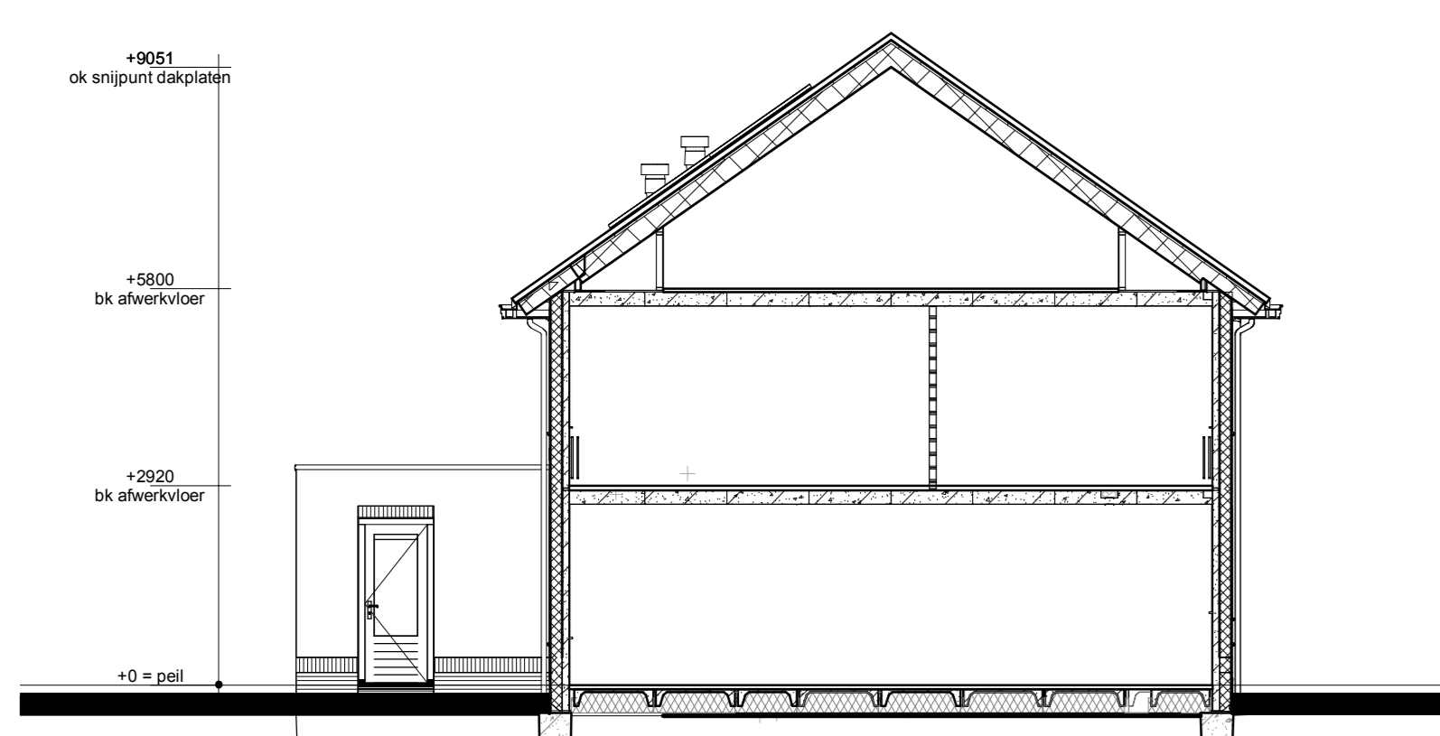
Doorsnede A1-A1
