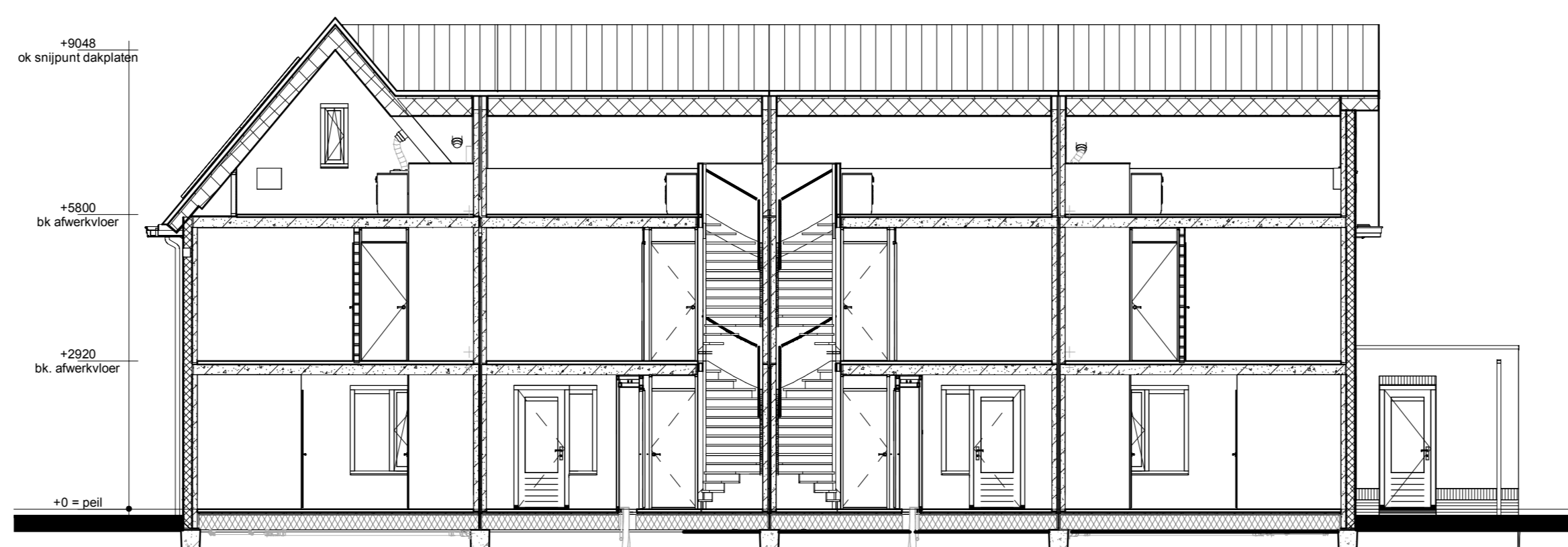
Doorsnede B1-B1
