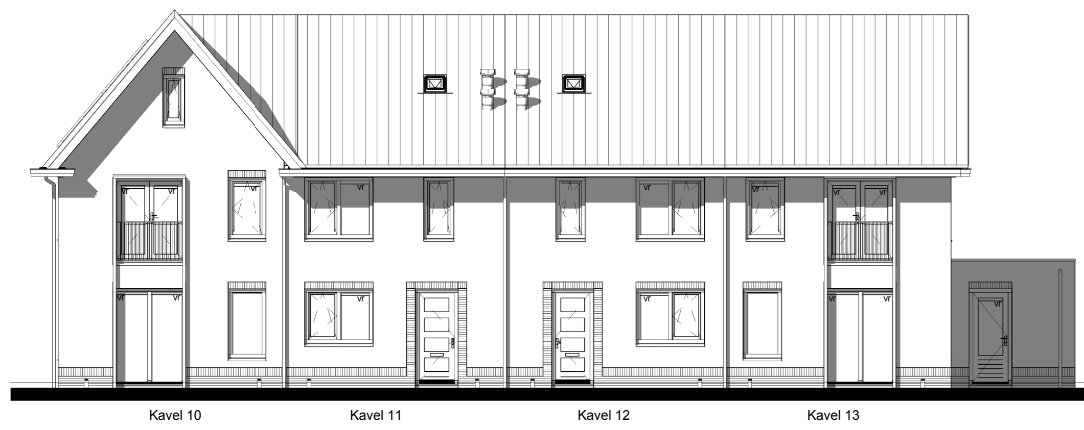
Voorgevel
