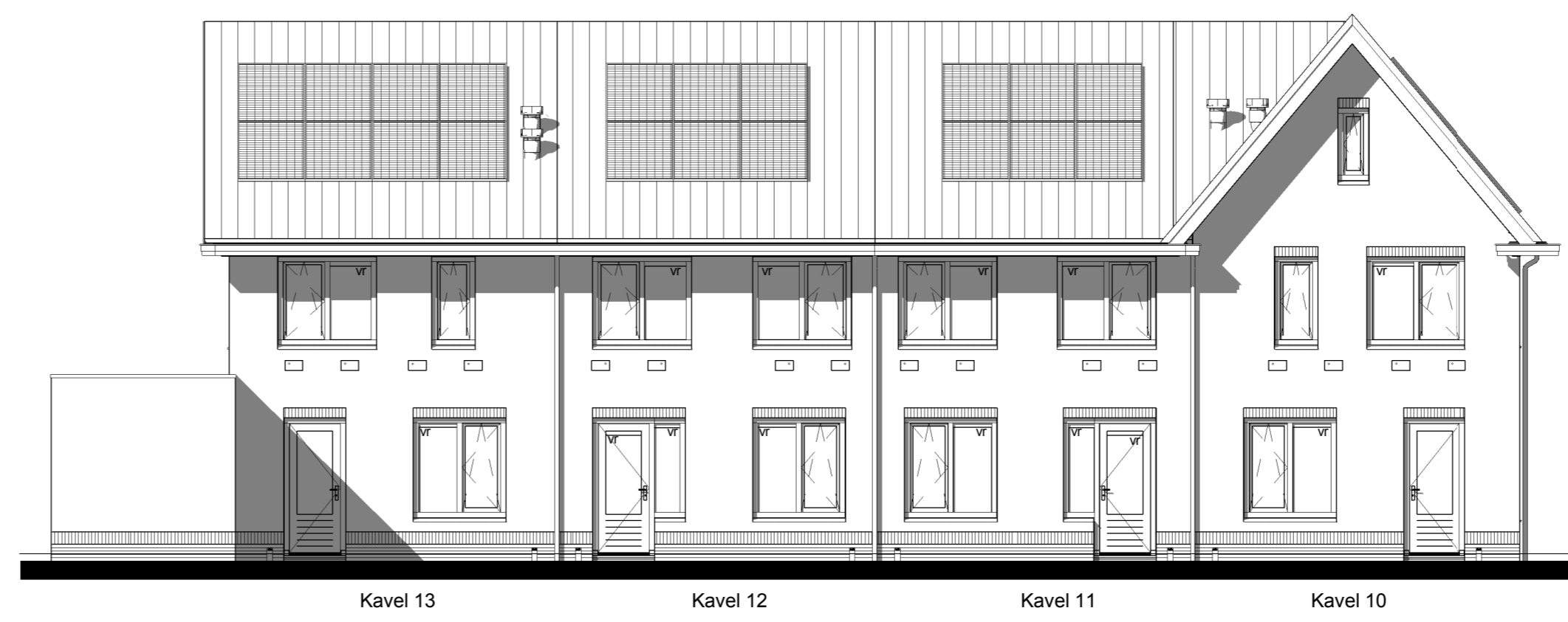
Achtergevel
