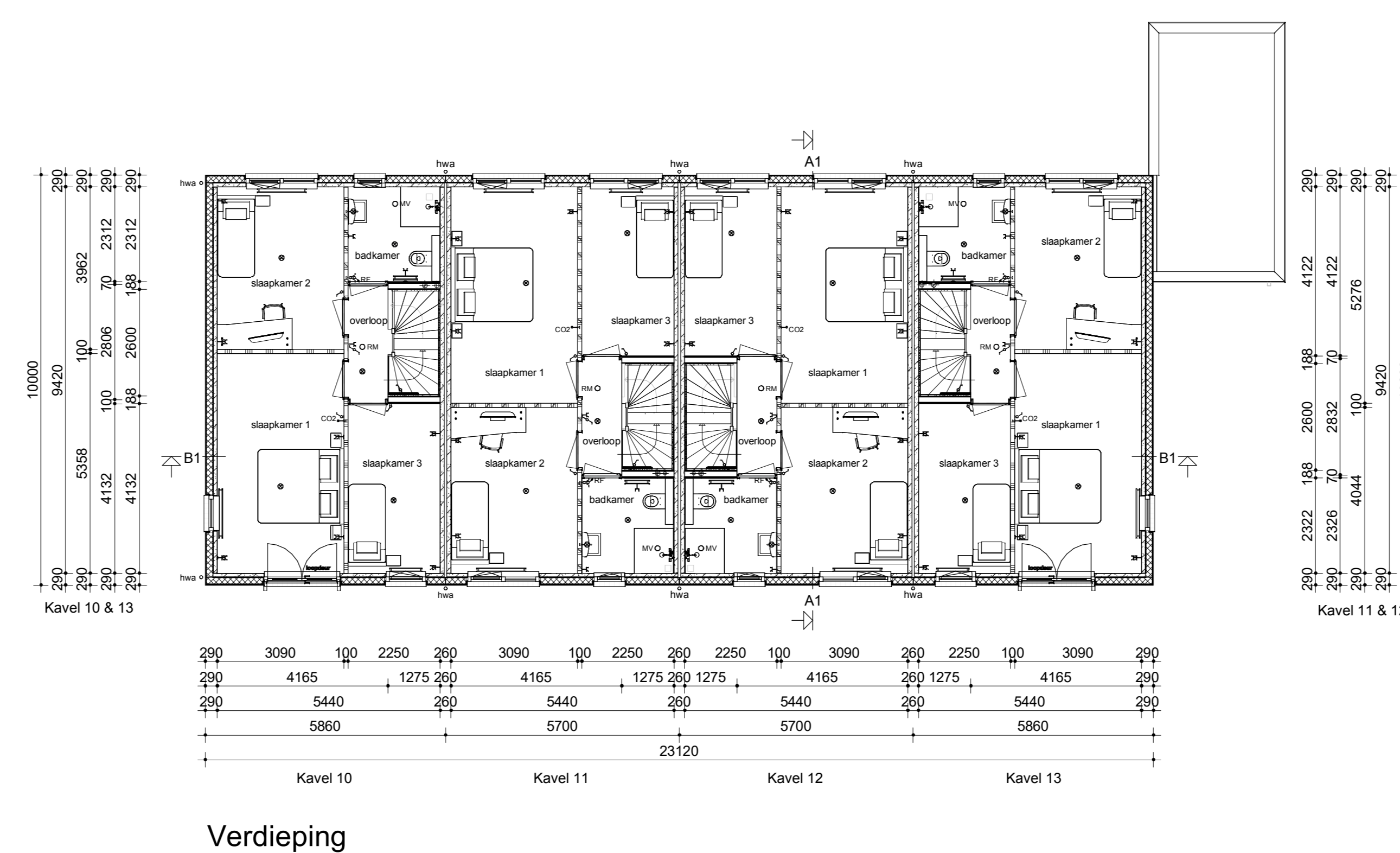
Verdieping
