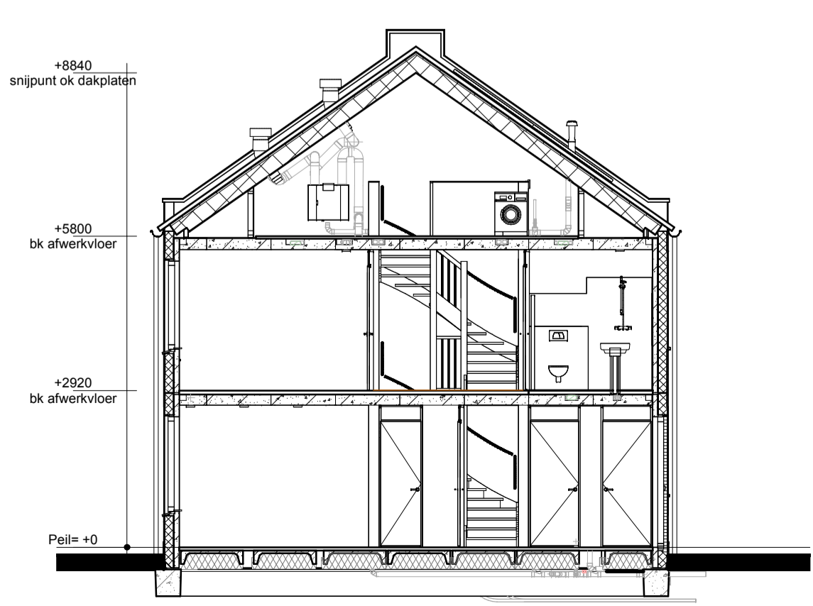
Doorsnede AA
